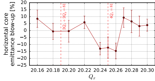
(d) Horizontal core emittance blow-up vs. horizontal tune
