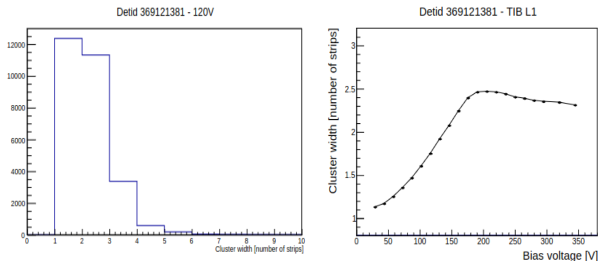
Figure 6.5: (Gauche) Distribution de la largeur de l'amas à l'étape 120 V du scan. (Droite) Courbe de la charge de l'amas en fonction de la tension de polarisation. Les deux figures proviennent du même scan d'août 2012 pour un module unique TIB L1. La tension de déplétion complète est d'environ 200 V.
