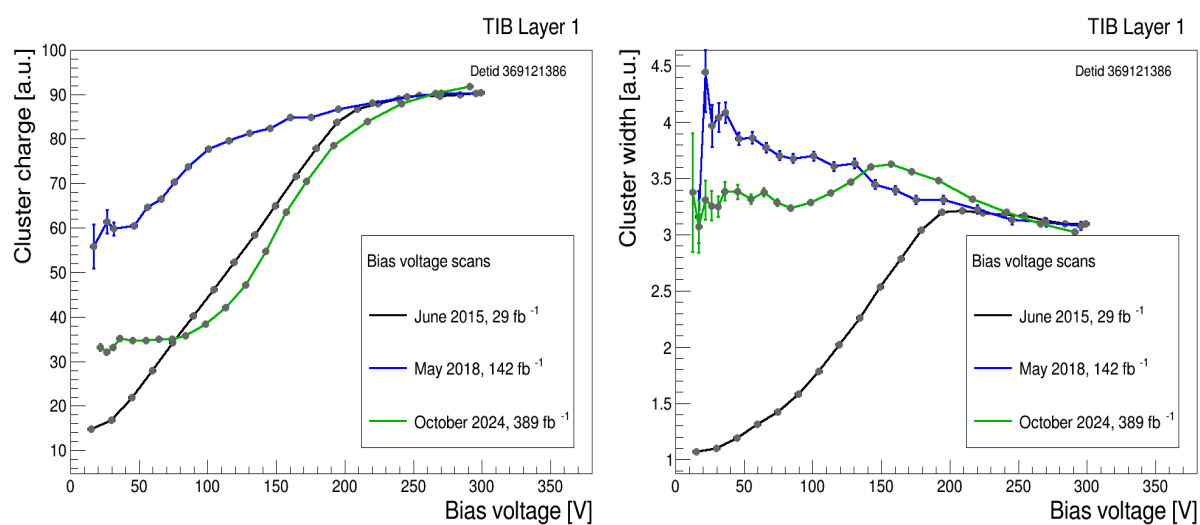
Figure 6.8: (Gauche) Courbes de la charge d'amas et (Droite) courbe de la largeur d'amas. Les scans ont été réalisés au début du Run 2 (2015), à la fin du Run 2 (2018) et au milieu des opérations du Run 3 (2024). Les graphiques sont montrés pour un module TIB L1.
