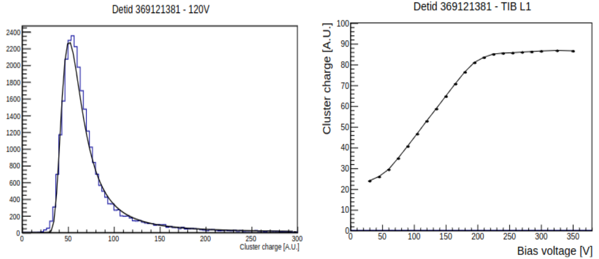
Figure 6.4: (Gauche) Distribution de la charge de l'amas à l'étape 120 V du scan. (Droite) Courbe de la charge de l'amas en fonction de la tension de polarisation. Les deux figures proviennent du même scan d'août 2012 pour un module unique TIB L1. La tension de déplétion complète est d'environ 200 V [85].
