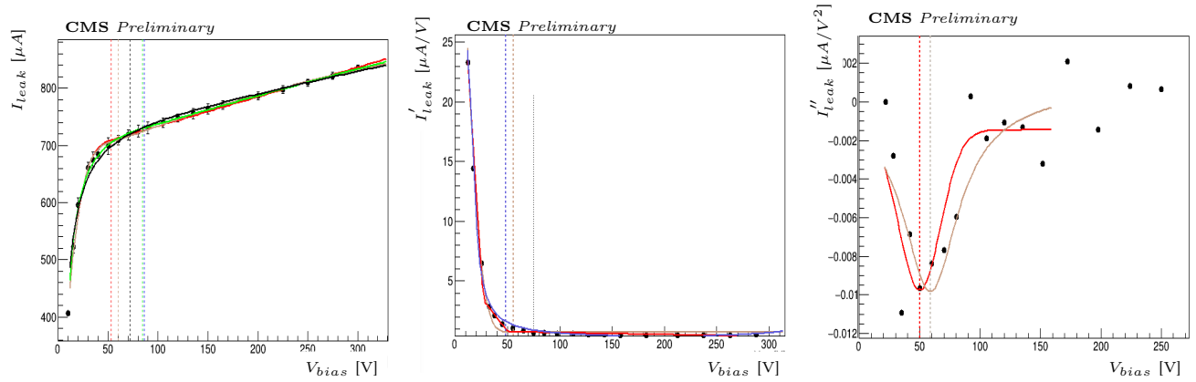
Figure 6.7: (Gauche) Courbe du courant de fuite avec les cinq ajustements différents. Les courbes rouge et marron représentent la sigmoïde avec les polynômes de premier et second ordre, respectivement. Les courbes bleue et verte correspondent à l'arctangente avec les polynômes de premier et second ordre, respectivement. La courbe noire est l'ajustement à usage général. (Milieu) Pente du courant de fuite en fonction de la tension de polarisation avec trois ajustements différents. L'ajustement gaussien/exponentiel est en marron, l'ajustement linéaire en rouge et l'ajustement à usage général en bleu. (Droite) Courbure du courant de fuite en fonction de la tension de polarisation avec deux ajustements différents. L'ajustement gaussien est en rouge tandis que la fonction à usage général est en marron. Les valeurs extraites de V_{FD} sont indiquées par les lignes verticales en pointillés. Les courbes sont montrées pour un module TIB L1 d'un scan de 2018 autour de l'inversion de type.
