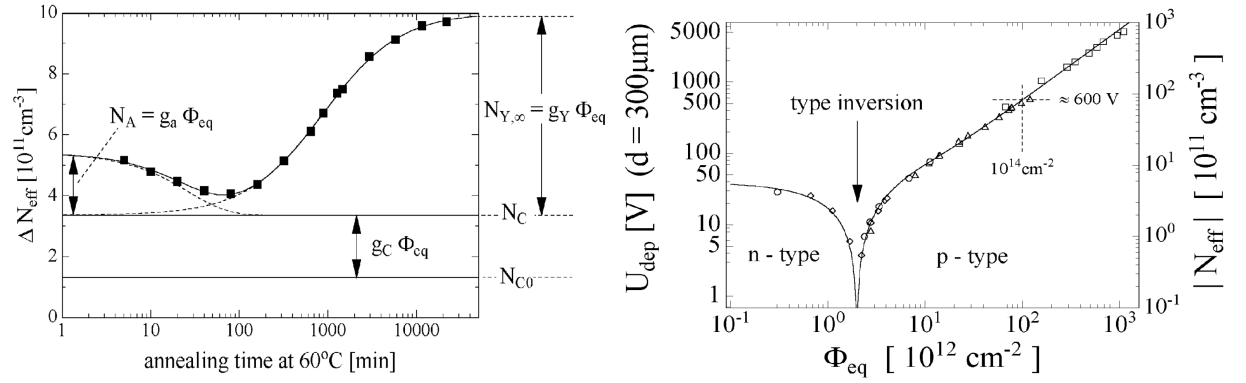
Figure 6.3: (Gauche) Variation de la concentration effective de dopage induite par l'irradiation, \Delta N_{eff} , à 6 °C. Le capteur a été exposé à une fluence de 1,4 \times 10^{13} \text{ cm}^{-2} [73]. (Droite) Variation de la tension de déplétion et de la valeur absolue de la concentration effective de dopage mesurées immédiatement après l'irradiation pour un capteur de 300 \mu\text{m} d'épaisseur [73].
