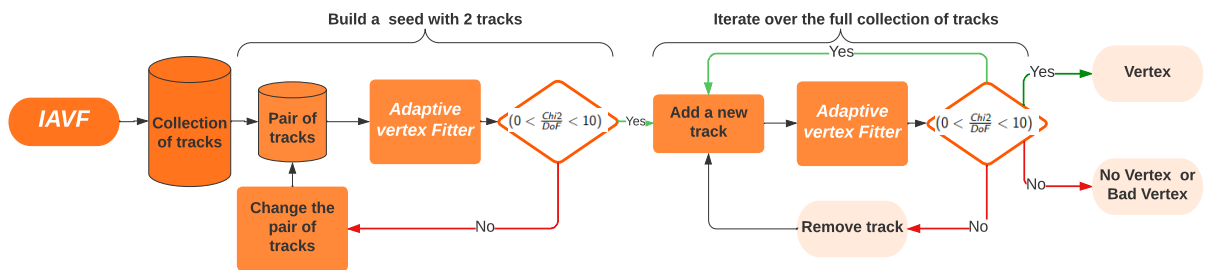
Figure 6.18: Représentation visuelle de l'IAVF.
