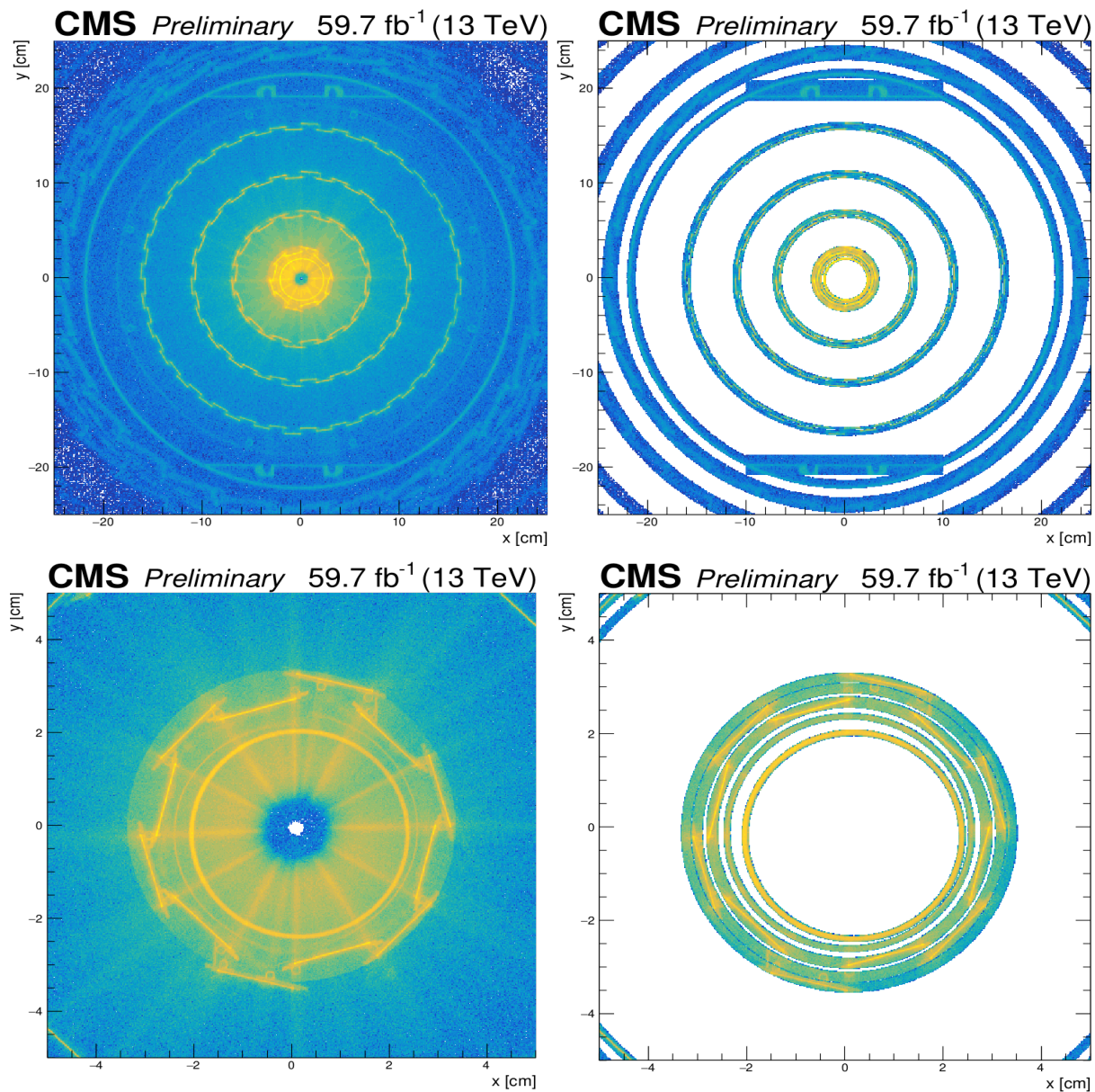
Figure 6.16: Distribution transverse des interactions secondaires dans le (haut) trajectographe et (bas) la couche interne de pixels pour l'échantillon de données \mu\mu de 2018 : (gauche) tous les vertex reconstruits, (droite) vertex exclus par veto. Pour plus de clarté, le vertex secondaire est demandé dans |\eta| < 1,4 .
