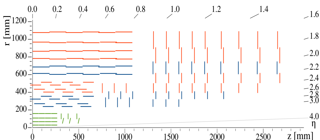
Figure 6.2: Schéma d'un quart du système de trajectographie de CMS en phase 1, dans le plan r - z . Le détecteur à pixels est représenté en vert, tandis que les modules de pistes simple face et double face sont figurés respectivement par des segments rouges et bleus [27].
