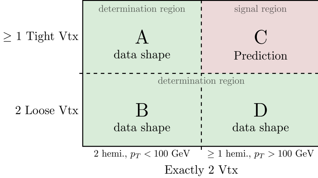
Figure 6.22: Vue schématique de la méthode d'estimation du bruit de fond. La forme du bruit de fond dans la région de signal C est définie à partir des données des régions A, B et D. L'évaluation bin par bin de la forme du fond dans la région de signal est définie par la relation n_C = n_A n_D / n_B .
