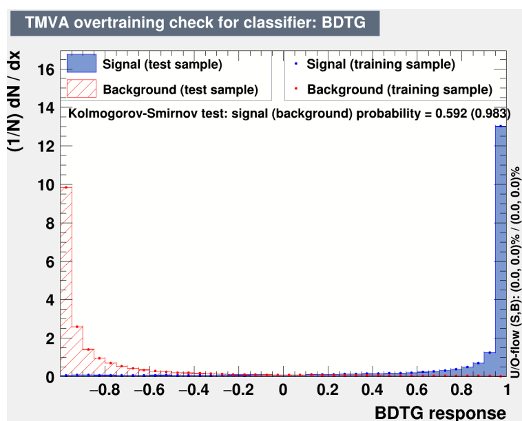
Figure 6.17: Test (histogrammes) et entraînement (points) du BDT des traces pour les traces de signal (issues des désintégrations de neutralinos) et les traces des bruits de fond.
