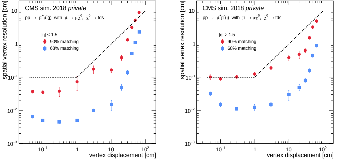
Figure 6.19: Résolution spatiale d'un vertex tight reconstruit dans les régions (gauche) centrale et (droite) bouchons en fonction de la distance de vol dans les événements MC de signal. Les deux distributions correspondent à 68% et 90% des vertex appariés entre vertex reconstruits et générés. Les valeurs sont obtenues à partir d'une collection d'échantillons de signal simulés dans les conditions MC de 2018. Les lignes pointillées représentent la résolution utilisée dans la procédure de fusion.
