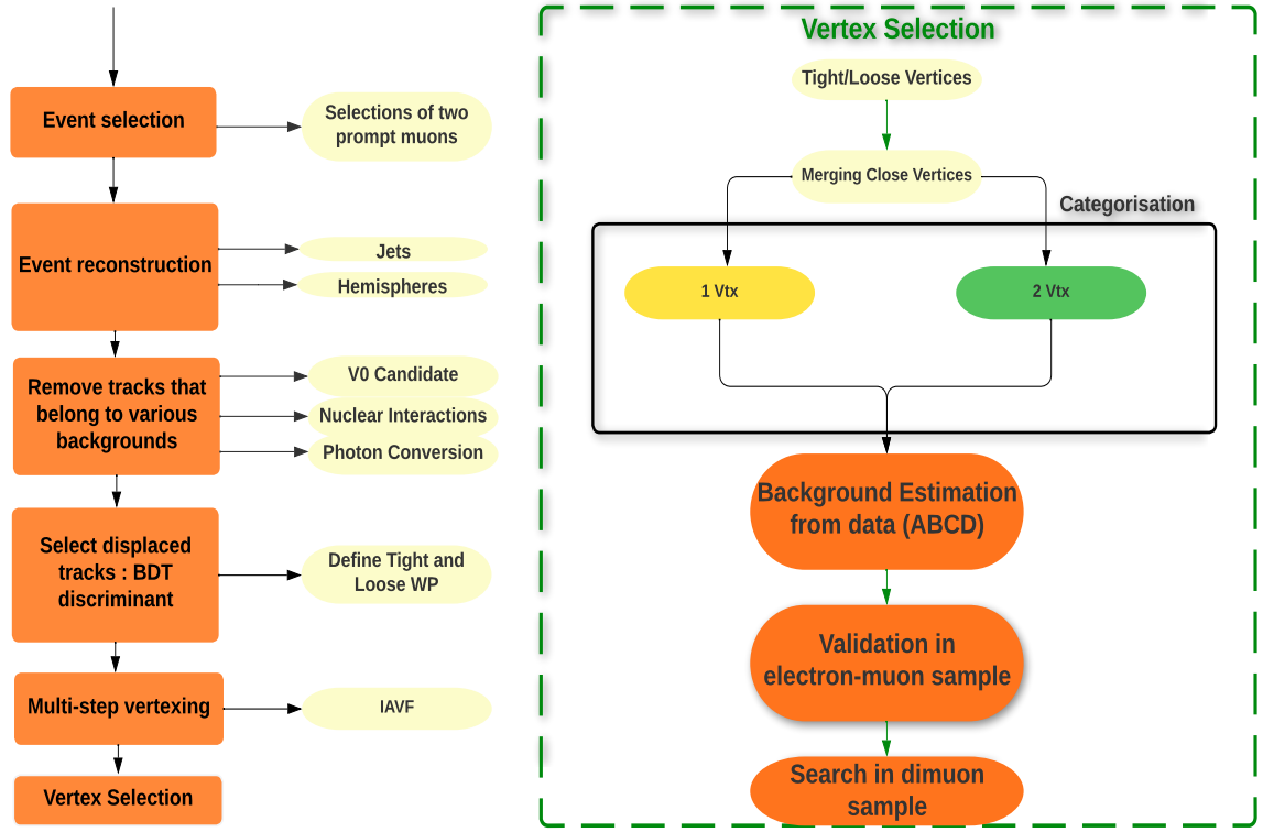
Figure 6.12: Schéma de la stratégie d'analyse.
