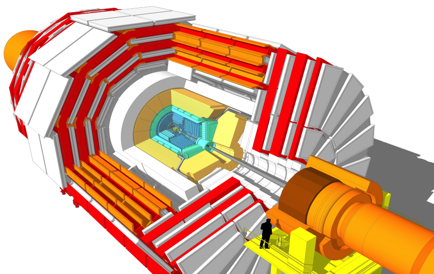
Figure 6.1: Image en coupe du détecteur CMS [24].
