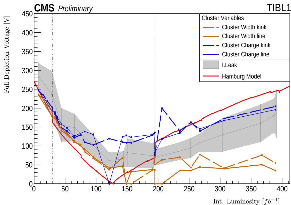
Figure 6.9: Tension de déplétion complète en fonction de la luminosité intégrée depuis le début des opérations du LHC jusqu'à la fin de 2024 pour les petits scans. Les valeurs extraites des trois observables sont montrées avec la largeur et la taille de l'amas affichées pour les deux méthodes d'extraction. La bande grise correspond aux extrêmes des dix fonctions d'ajustement différentes des courbes de courant de fuite. Le comportement prédit par le modèle de Hambourg est indiqué en rouge. Les courbes de clusters atteignent 0 lorsque la méthode d'extraction n'a pas pu converger. Les lignes verticales en pointillés noirs indiquent les LS1 ( 30 fb^{-1} ) et LS2 ( 200 fb^{-1} ). Le dernier point de données correspond au dernier scan avant les opérations de 2025. L'effet de bascule observé autour de LS2 n'est pas clairement compris. L'incertitude sur les courbes des amas est d'environ 20–30 V, liée aux limitations statistiques des petits scans.
