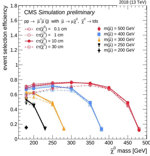
Figure 6.15: Efficacité des événements de signal à passer la sélection d'événement en fonction des masses du neutralino et du smuon ainsi que de la durée de vie du neutralino dans les conditions MC de 2018.
