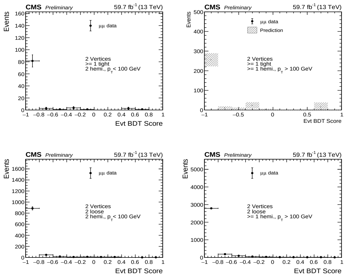
Figure 6.25: Méthode d'estimation du bruit de fond appliquée à l'échantillon \mu\mu de 2018, avec la région de signal (SR) masquée, en tenant compte de la correction associée à la corrélation.
