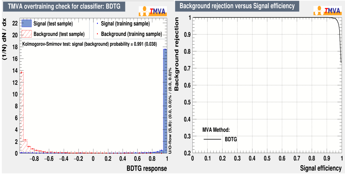
Figure 6.23: (Gauche) Distributions d'entraînement et de test pour les vertex (bleu) signal et (rouge) fond. (Droite) Courbe ROC associée.
