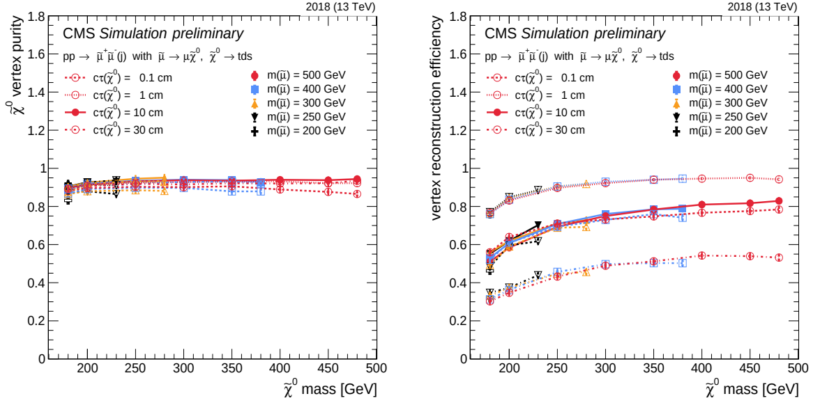
Figure 6.21: La (gauche) pureté et (droite) efficacité des vertex déplacés tight reconstruits en fonction des masses du neutralino et du smuon pour différents c\tau_{\tilde{\chi}} du neutralino dans les conditions MC de 2018.
