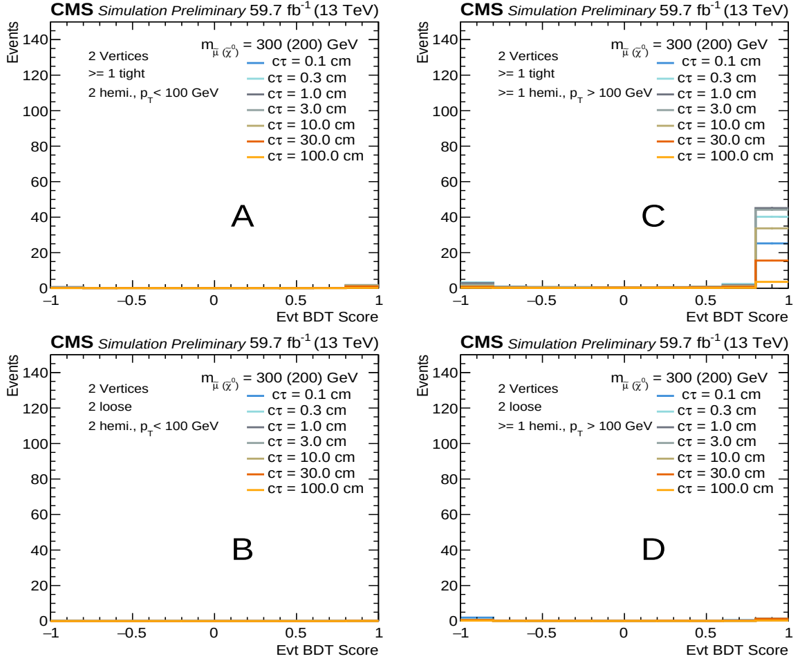
Figure 6.24: Score BDT de l'événement pour deux vertex dans des événements de signal avec S_{m_{\tilde{\chi}_0^1}}^{m_{\tilde{\mu}}} = S_{200}^{300} dans les conditions MC de 2018 pour différentes valeurs de c\tau_{\tilde{\chi}} .
