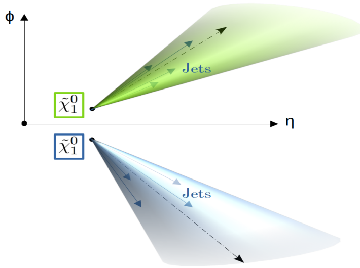
Figure 6.13: Schéma de la désintégration des deux neutralinos. Les flèches noires en pointillées indiquent la direction de l'impulsion du neutralino généré.
