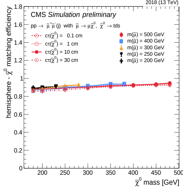
Figure 6.14: Efficacité à associer l'axe de l'hémisphère reconstruit à la direction du neutralino généré le plus proche ( \Delta R < 1,5 ) en fonction des masses du neutralino et du smuon ainsi que de la durée de vie du neutralino dans les conditions MC de 2018.
