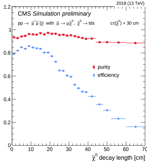
Figure 6.20: Efficacité de reconstruction des vertex tight (bleu) et pureté (rouge) en fonction de la longueur de désintégration du neutralino. Les événements de signal sont simulés dans les conditions de 2018 pour une large gamme de masses de smuon et de neutralino, avec un c\tau_{\tilde{\chi}} du neutralino de 30 cm.
