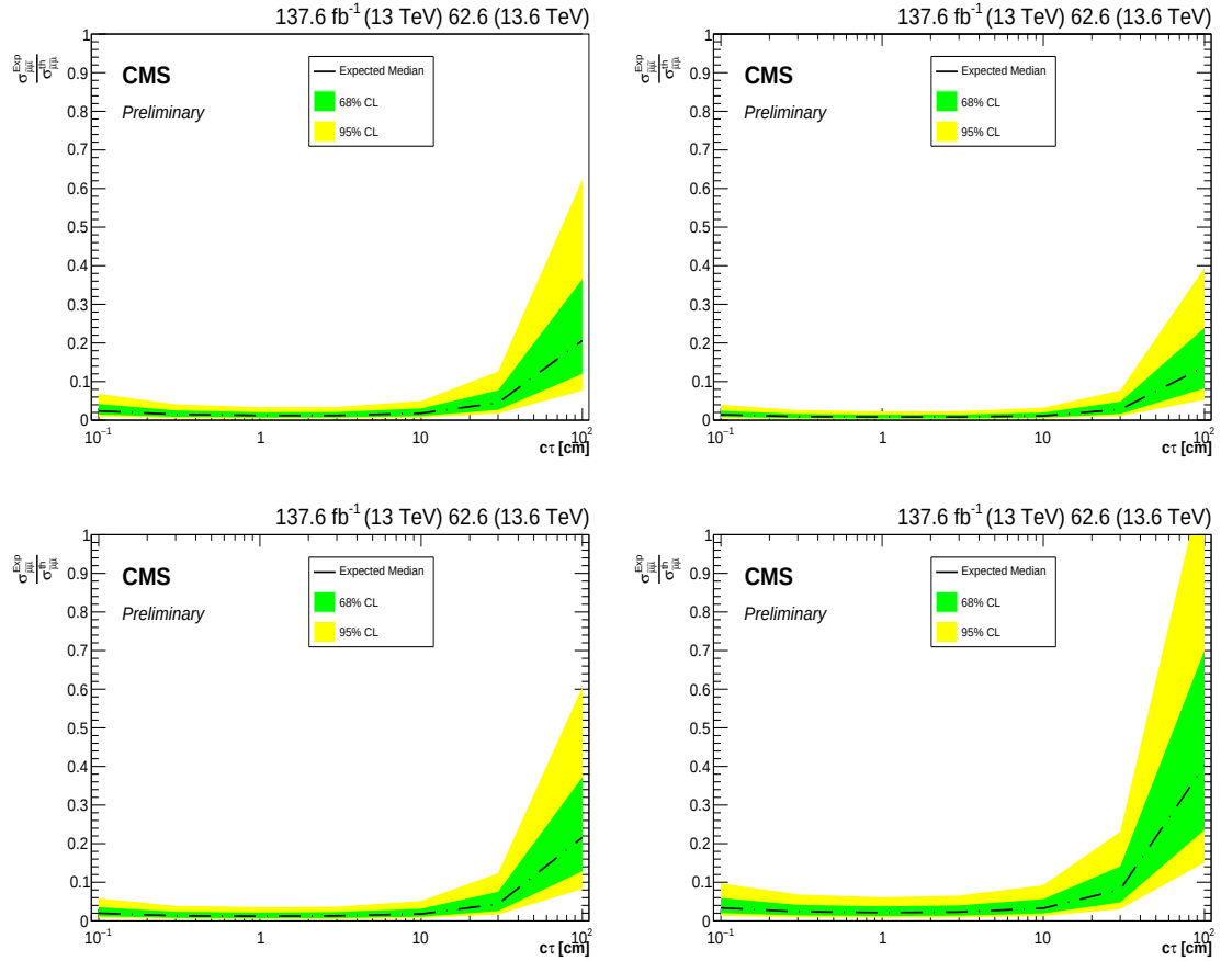
Figure 6.26: \sigma_{\tilde{\mu}\tilde{\mu}} \times B_r(\tilde{\mu} \rightarrow \mu\tilde{\chi}^{01})^2 en supposant différentes combinaisons de masses entre le smuon et le neutralino S^{m\tilde{\mu}}m_{\tilde{\chi}_0^1} : (haut gauche) S^{200}180 , (haut droite) S^{250}200 , (bas gauche) S^{300}200 , (bas droite) S^{350}200 . Les échantillons de signal pour lesquels le rapport des sections efficaces est inférieur à 1 sont exclus.
