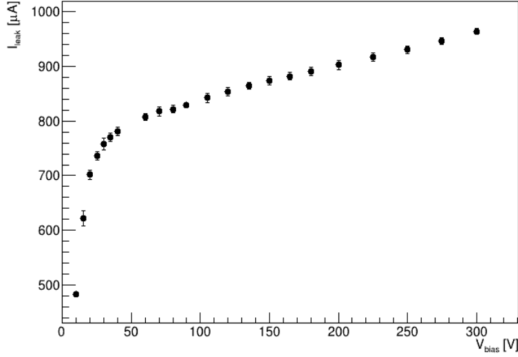
Figure 6.6: Distribution du courant de fuite en fonction de la tension de polarisation d'un module TIB L1 lors d'un scan de 2018, proche de l'inversion de type du module [85].
