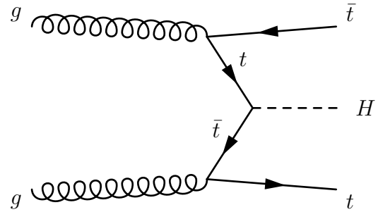
(d) t\bar{t} Fusion
