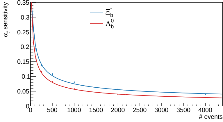
Figura R.6: Sensibilidad a la medida de la polarización del fotón en función del número de eventos de señal para los canales de desintegración \Lambda_b^0 \rightarrow \Lambda \gamma (rojo) y \Xi_b^- \rightarrow \Xi^- \gamma (azul). La distribución se ajusta a la función 1/\sqrt{N} para ver mejor su tendencia.
