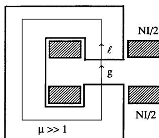
FIG. 6.2 – Ampère-tours dans un dipôle
