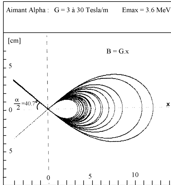
FIG. 2.3 – Trajectoire de particules de différentes énergies dans un aimant alpha.
