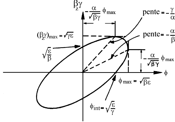
FIG. 3.3 – Paramètres de l'ellipse pour l'espace des phases longitudinal.
