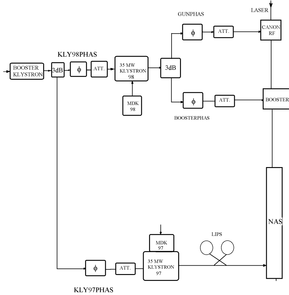
FIG. 7.1 – Distribution RF dans le CTF.
