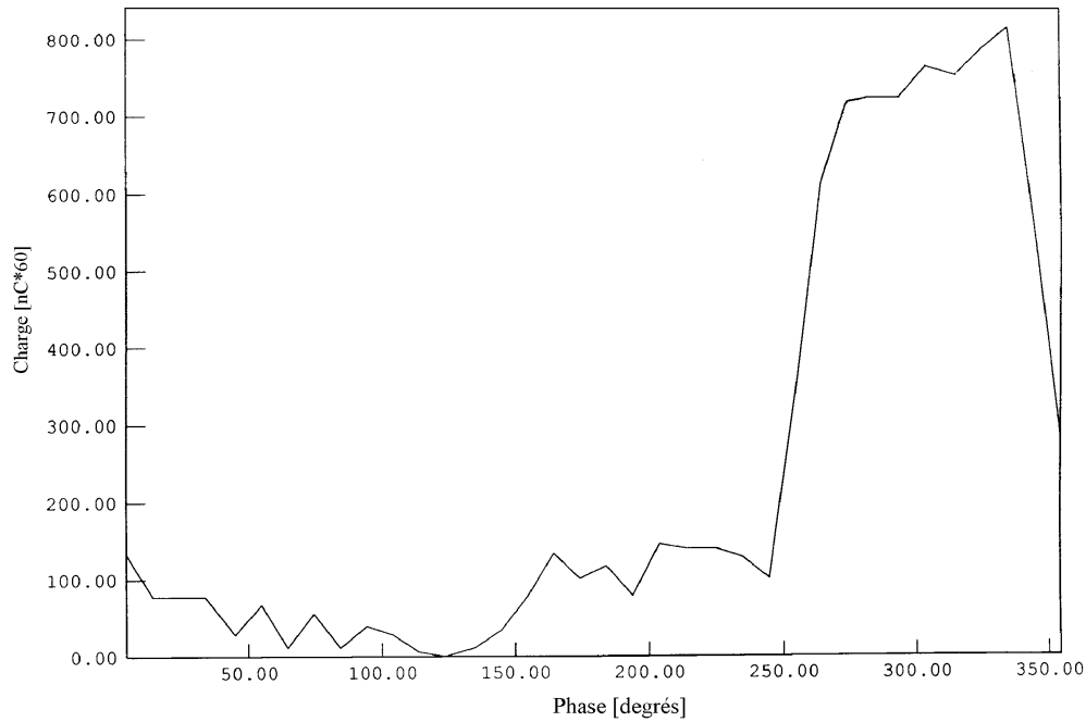
FIG. 7.7 – Charge transmise à la sortie du booster en fonction de la phase de l'onde RF dans le canon.
