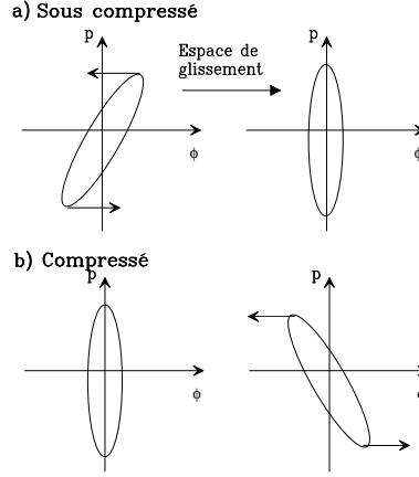
FIG. D.1 – Evolution de l'espace de phases à partir de la sortie du compresseur.
