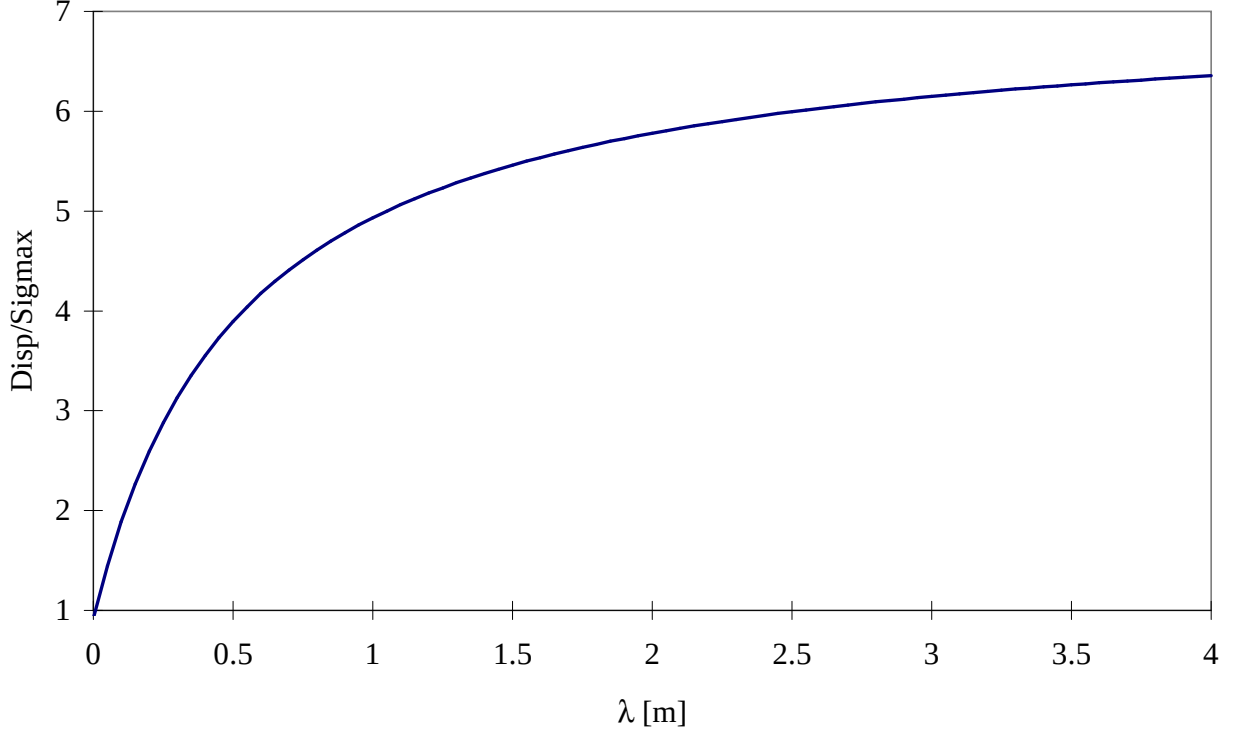
FIG. 3.9 – Rapport Disp/sigma_x en fonction de \lambda .
