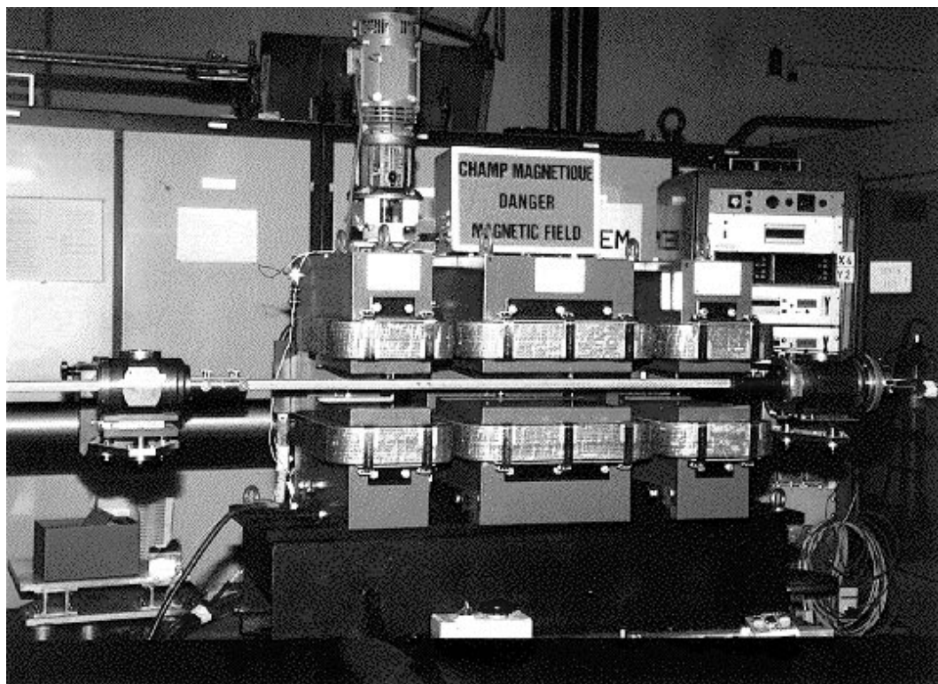
FIG. 6.9 – Le compresseur de paquets sur son banc de mesures magnétiques
