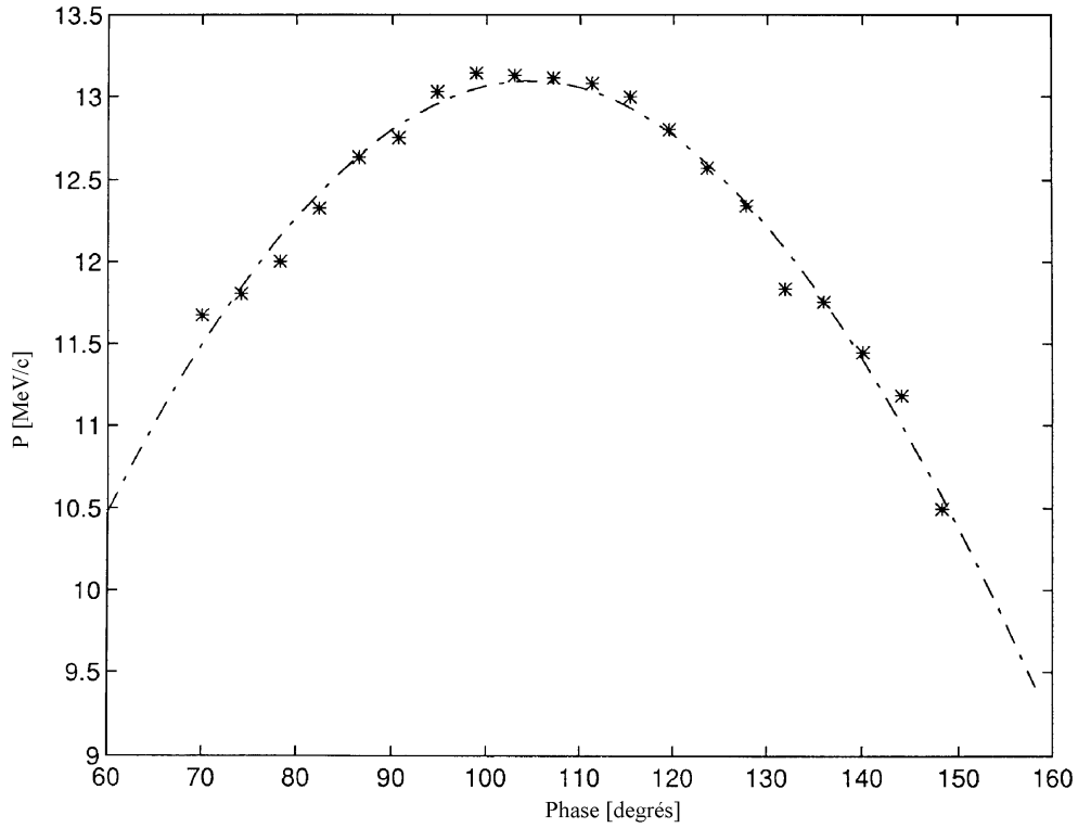
FIG. 7.8 – Energie du faisceau en fonction de la phase du booster.
