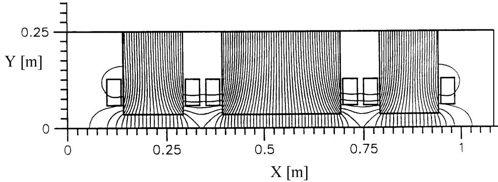
FIG. 6.6 – Lignes de flux magnétique
