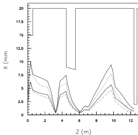
(d) Enveloppes verticales à 5 nC
