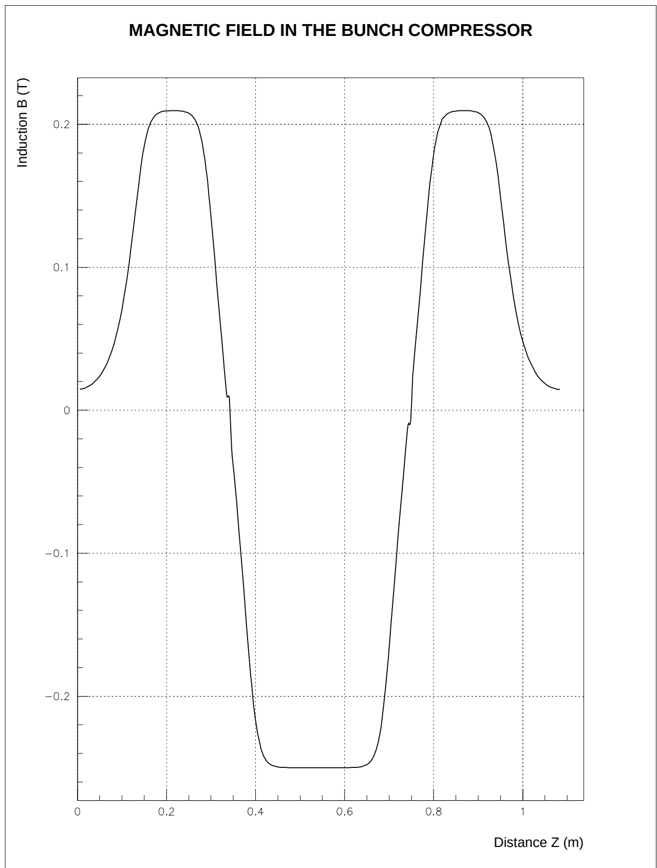
FIG. 6.7 – Profil longitudinal du champ magnétique. (Simulation)
