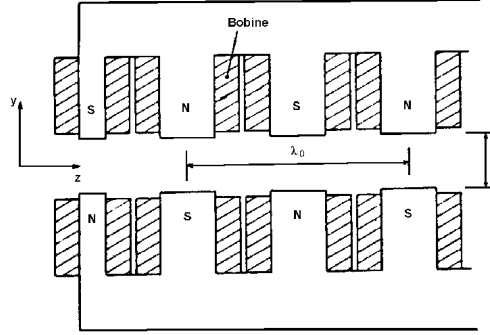
FIG. 2.2 – Géométrie d'un onduleur plan à électroaimants
