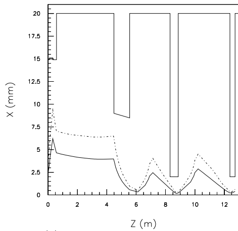
(e) 1 nC avec des impulsions laser de 3 ps rms
