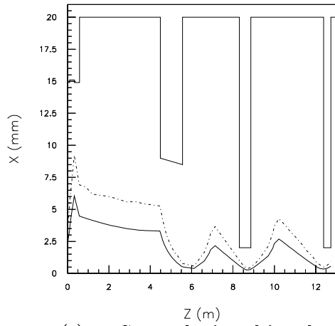
(c) 1 nC avec des impulsions laser de 8 ps rms
