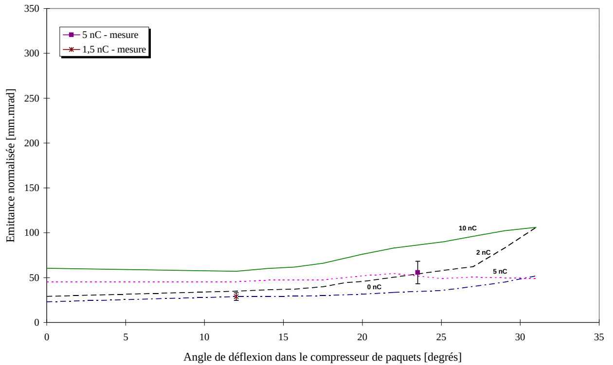
(b) Emittance normalisée verticale
