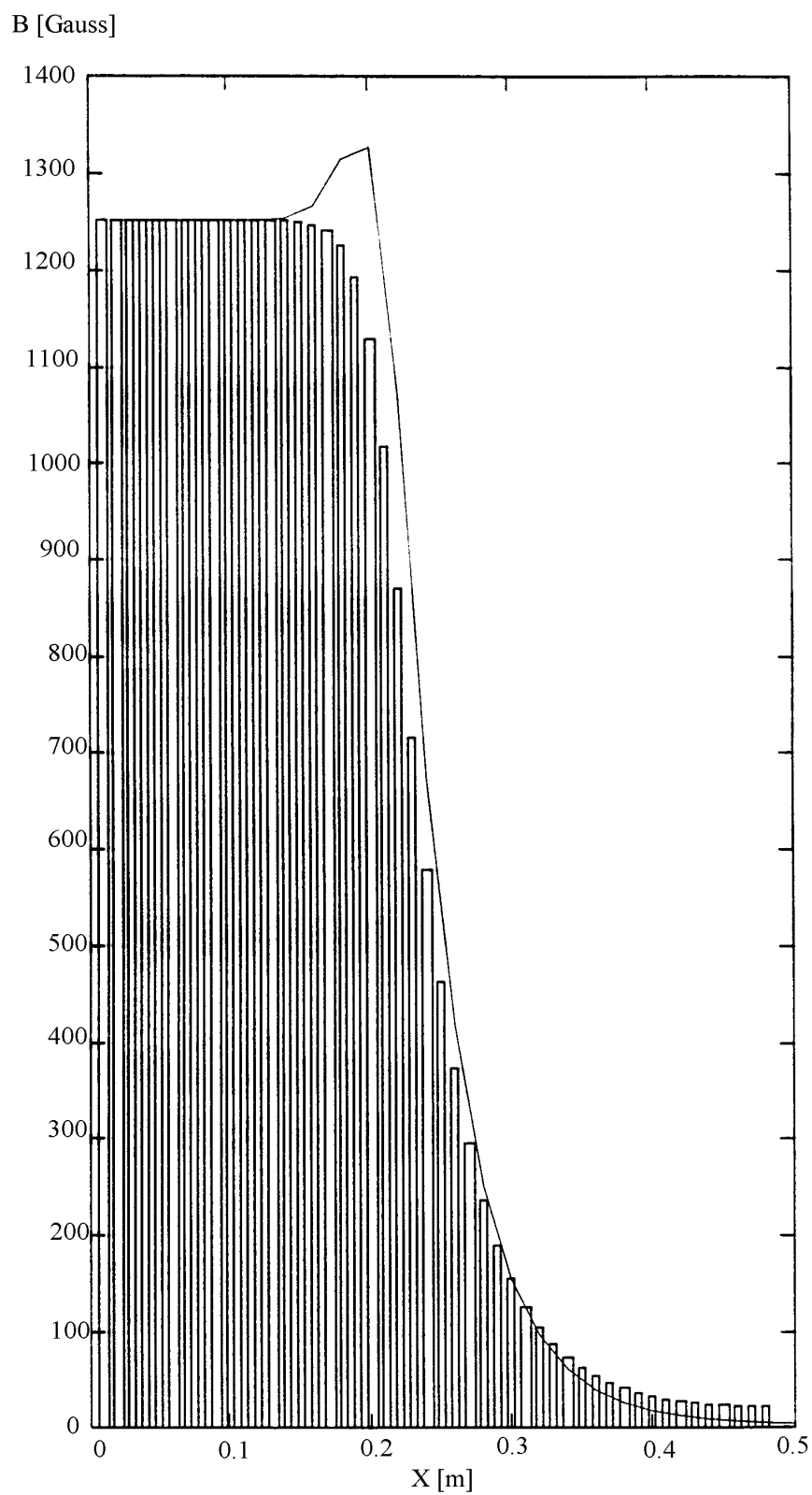
FIG. 6.5 – Superposition des champs magnétiques mesuré et calculé.
