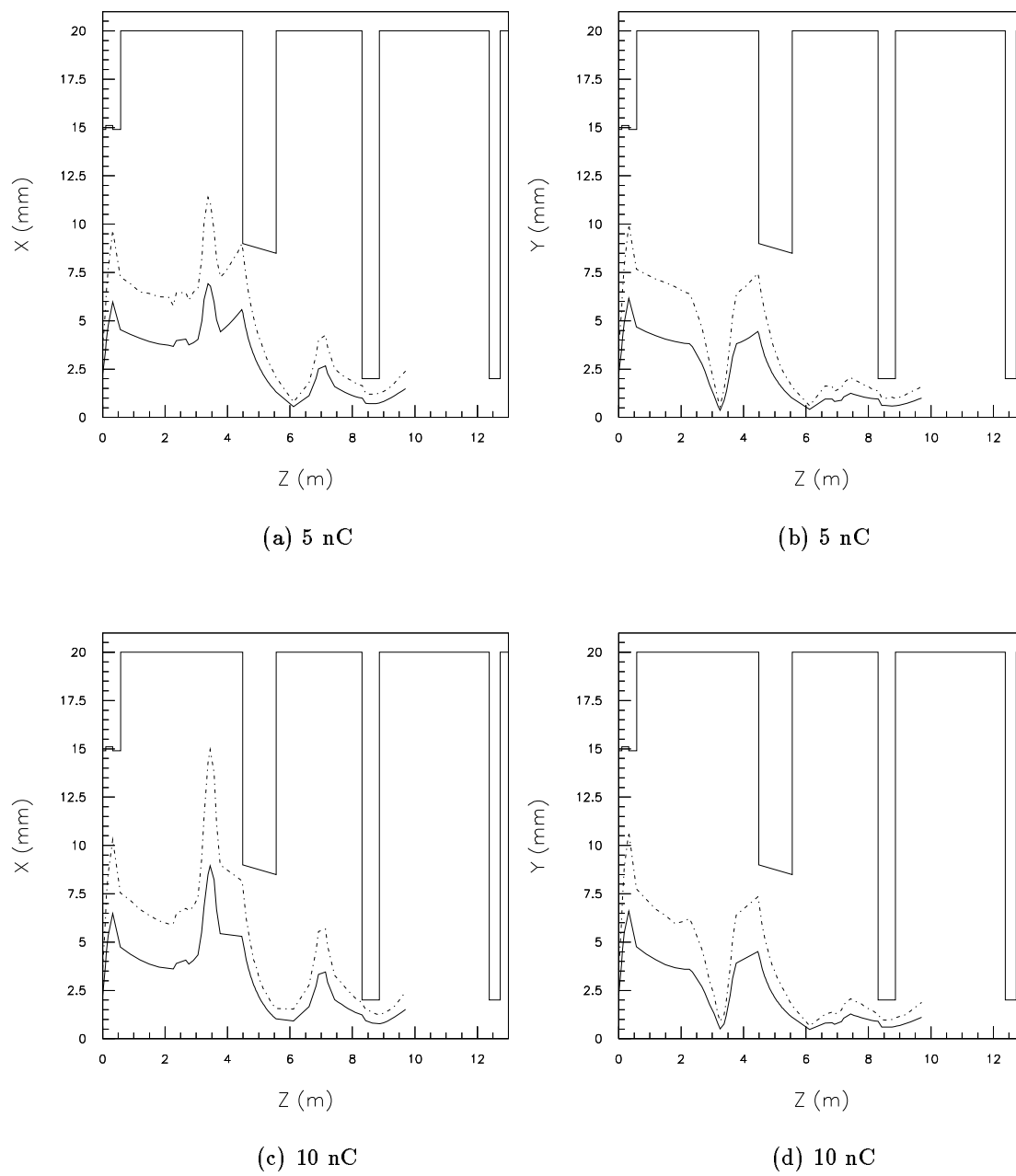
FIG. 4.22 – Enveloppes pour les tests des BPM à 5 nC et 10 nC. (...) : 90% de particules. (-) : valeur rms.
