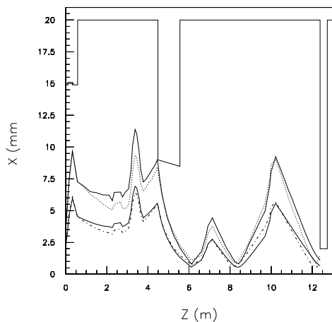
(c) Enveloppes horizontales à 5 nC
