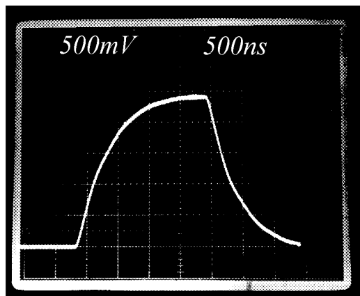
FIG. 7.2 – Etablissement du champ électrique dans la première demi-cellule du canon (2,5 V représentent 100 MV/m).
