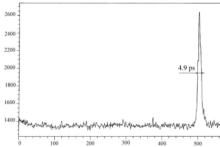
(b) Après compression
