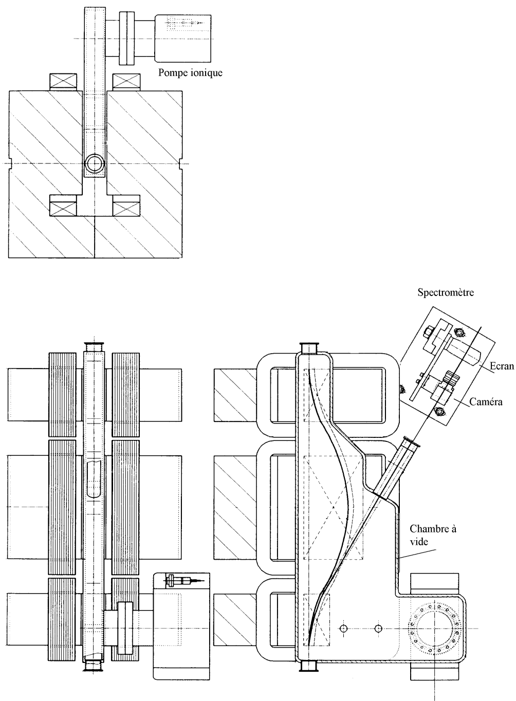
FIG. 6.10 – Dessin d'ensemble du compresseur de paquets avec sa chambre à vide.
