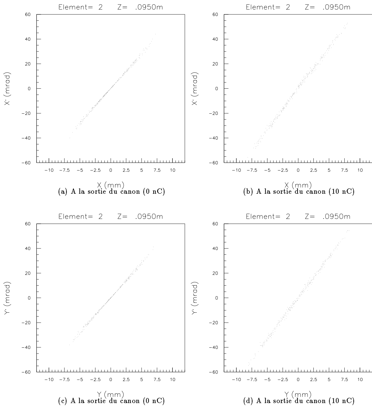
FIG. 4.10 – Espace des phases transversal à la sortie du canon pour 0 et 10 nC.
