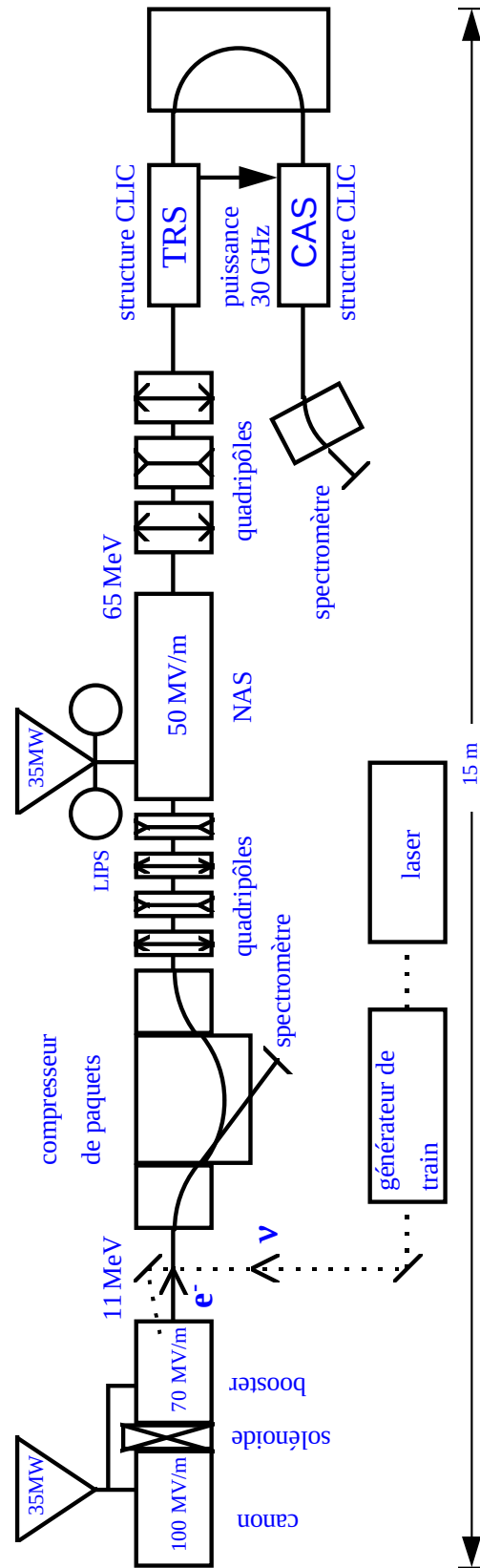
FIG. 1.2 – Dessin d'ensemble du CTF 1995.
