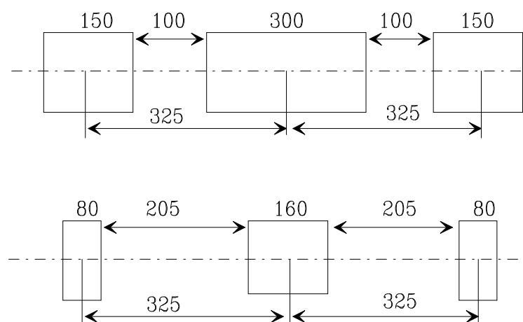
FIG. 6.8 – Les deux optiques utilisées avec le code TRANSPORT .
