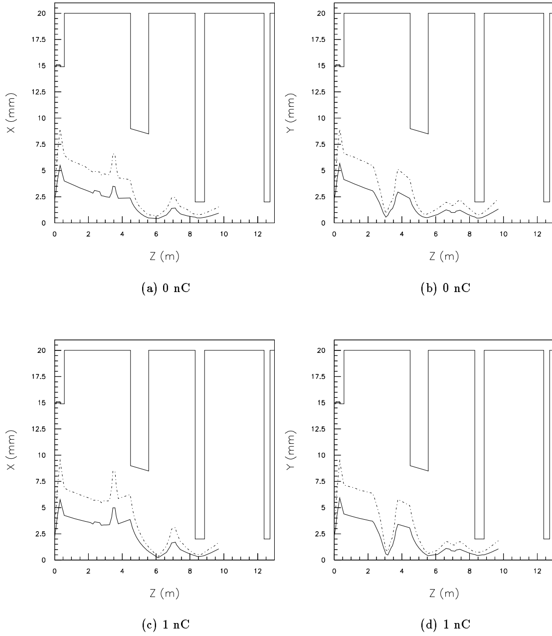
FIG. 4.21 – Envelopes pour les tests des BPM à 0 nC et 1 nC.
