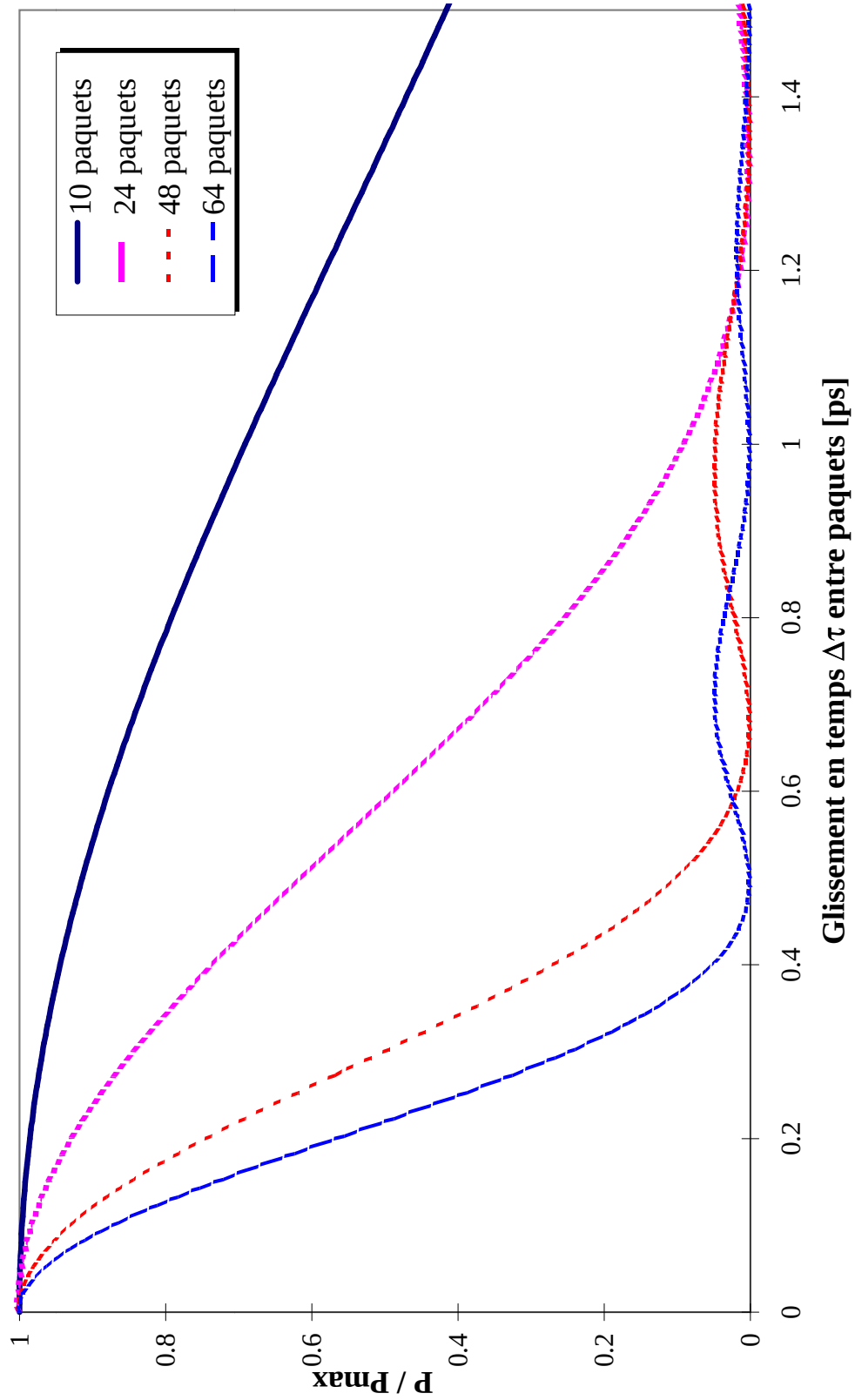
FIG. 5.3 – Production relative de puissance à 30 GHz créée par des trains dont les paquets sont espacés régulièrement d'une quantité \Delta\tau par rapport à \lambda_{30\text{GHz}} .
