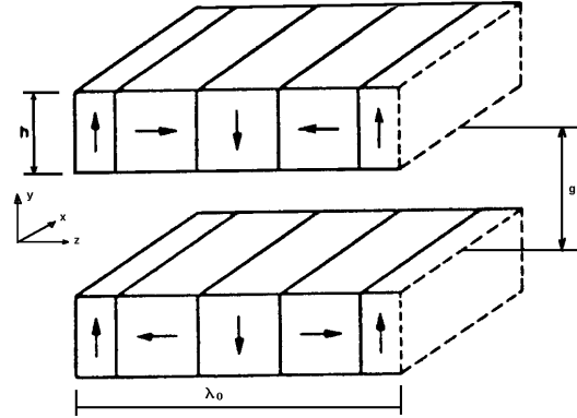
FIG. 2.1 – Géométrie d'un onduleur plan à aimants permanents
