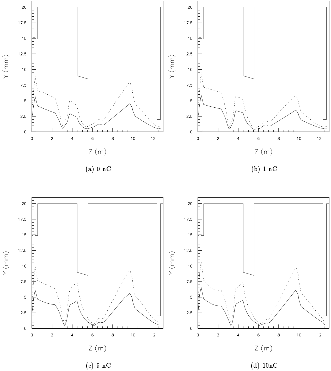
FIG. 4.4 – Enveloppes verticales pour une transmission maximale.
