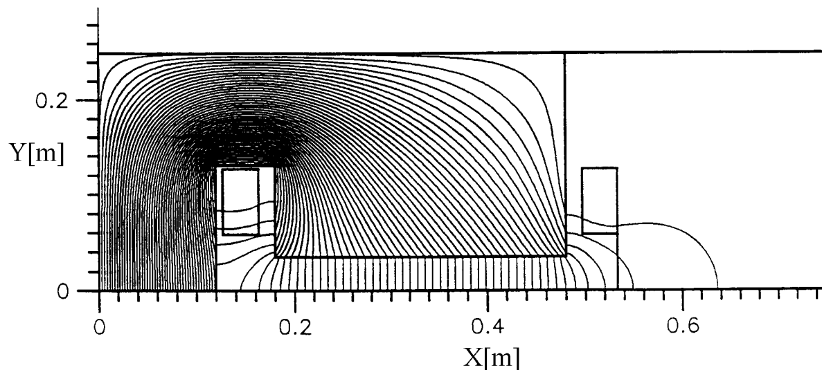
FIG. 6.1 – Lignes de flux magnétique. Coupe transversale.
