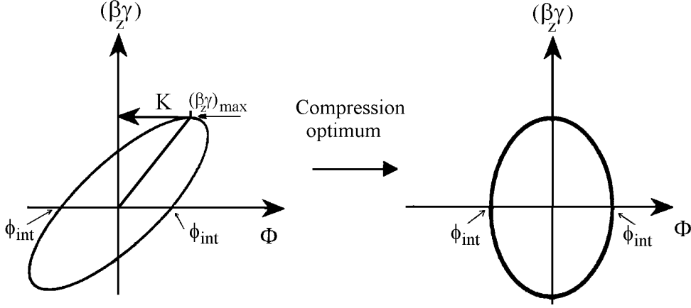
FIG. 3.2 – Processus de compression dans (\phi, (\beta_z \gamma))
