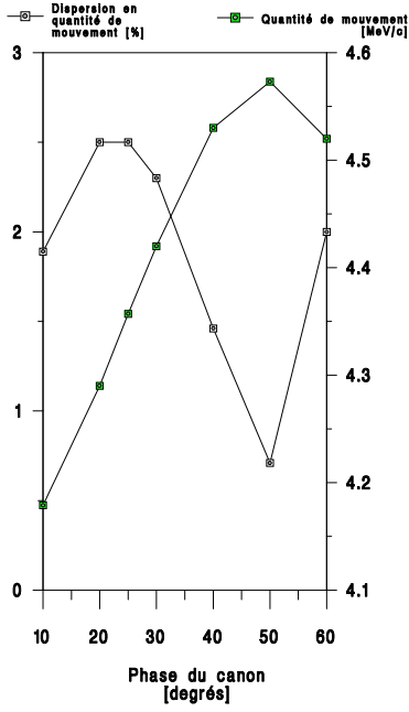
(a) A la sortie du canon
