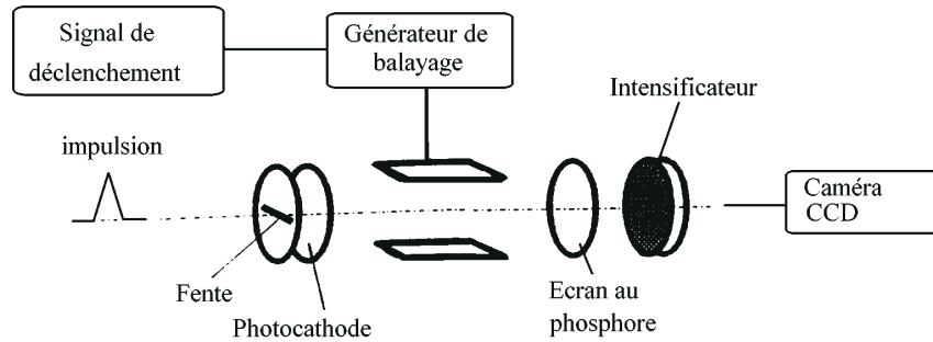
FIG. 7.6 – Fonctionnement d'une caméra à balayage rapide
