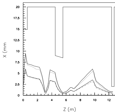
(b) Enveloppes verticales à 1 nC
