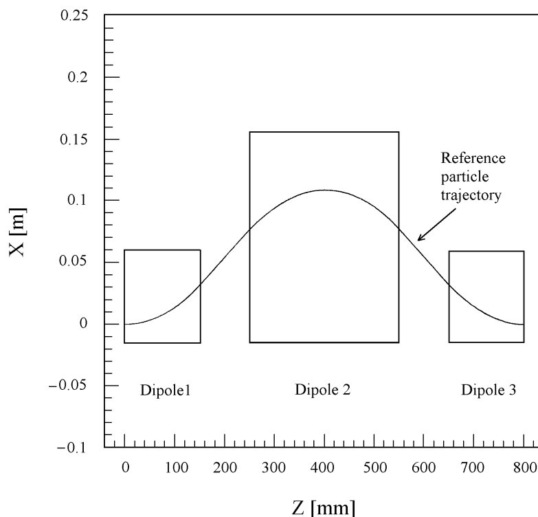
FIG. 3.8 – Trajectoire centrale dans le compresseur de paquets.
