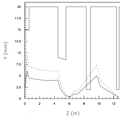
(f) 1 nC avec des impulsions laser de 3 ps rms
