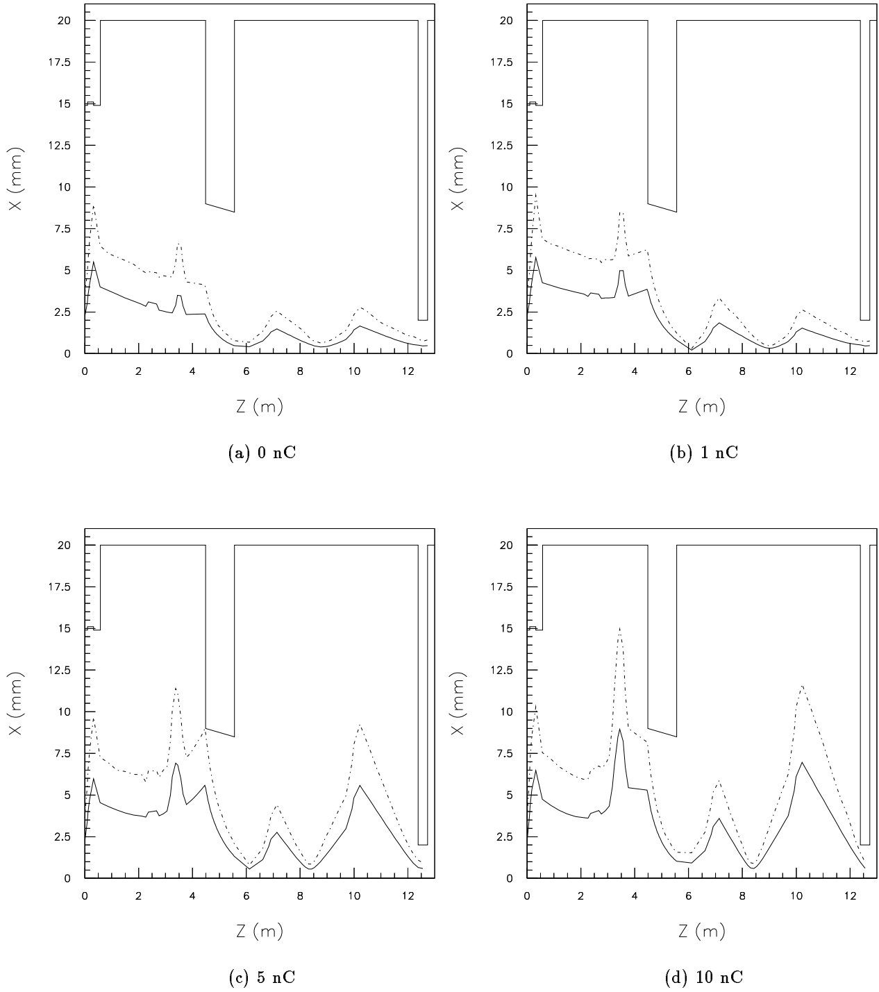
FIG. 4.3 – Envelopes horizontales pour une transmission maximale.
