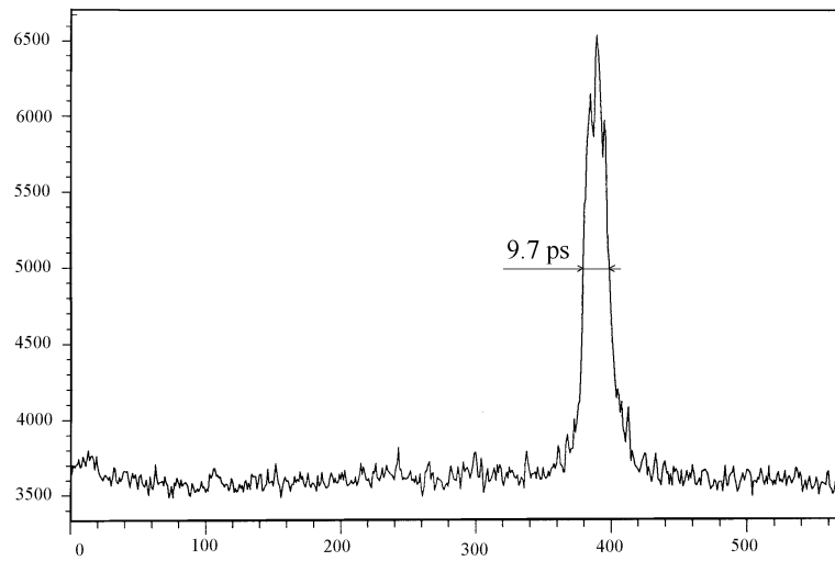
(a) Avant compression
