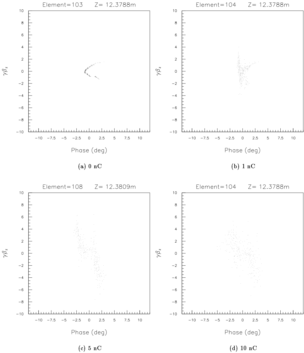
FIG. 4.9 – Espace des phases longitudinal à l'entrée de TRS pour différentes charges.
