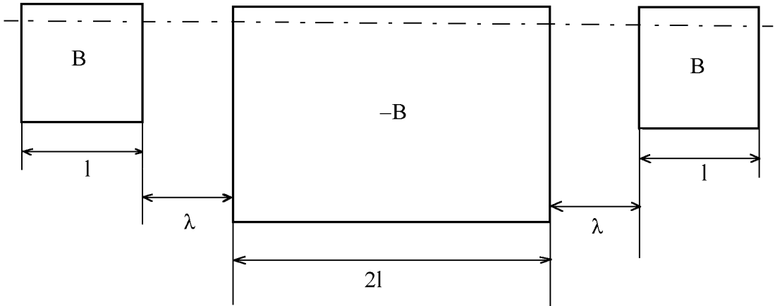
FIG. 3.7 – Longueurs et champs magnétiques pour un système de compresseur de paquets à symétrie centrale.
