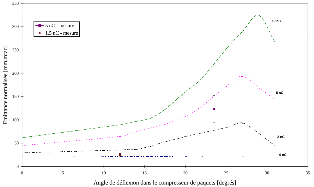
(a) Emittance normalisée horizontale
