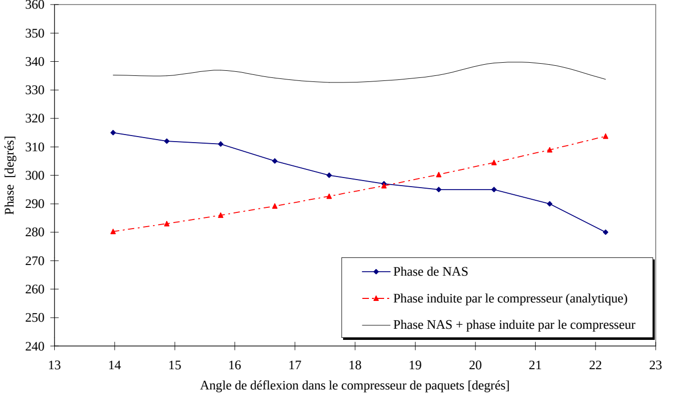
FIG. 7.9 – Comparaison entre l'évolution de la phase du faisceau calculée analytiquement et la phase de NAS mesurée en fonction de l'angle de déflexion dans le compresseur de paquets. Les phases sont relatives.
