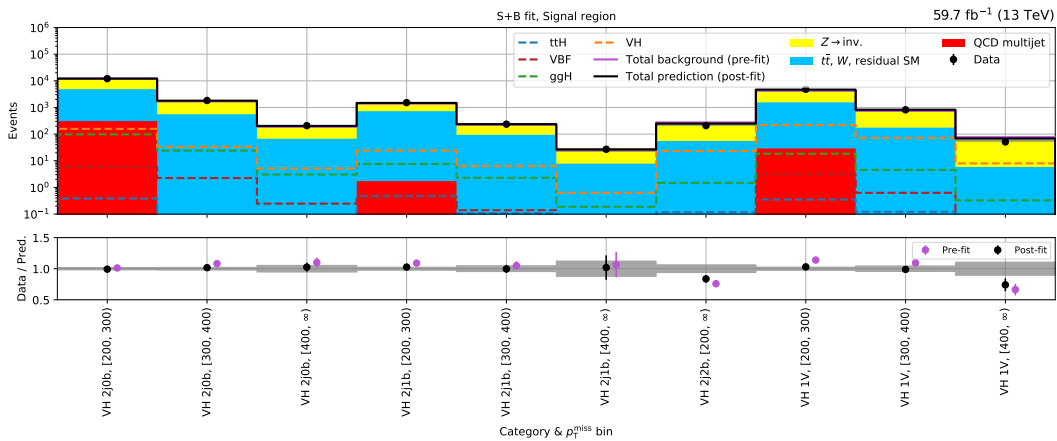
(c) VH —2018
