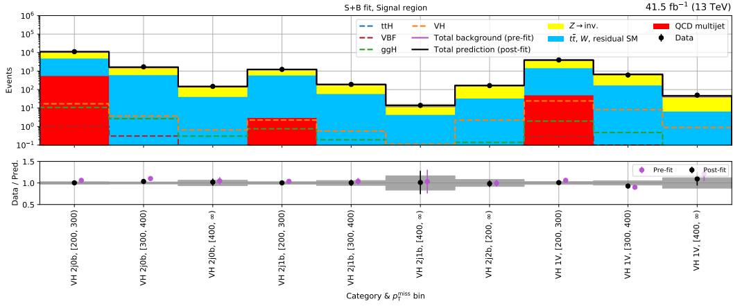
(b) VH —2017
