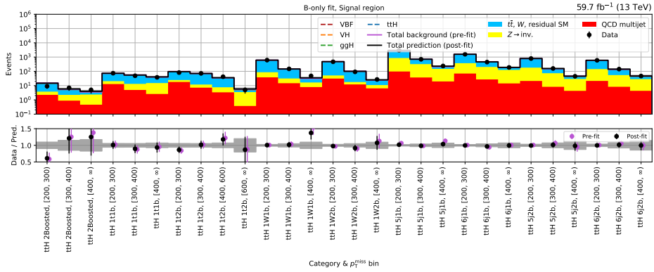
(c) t\bar{t}H —2018
