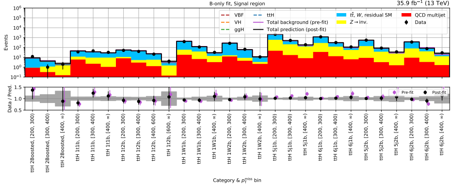
(a) t\bar{t}H —2016
