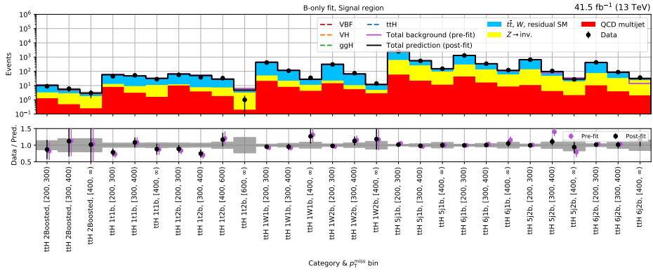
(b) t\bar{t}H —2017
