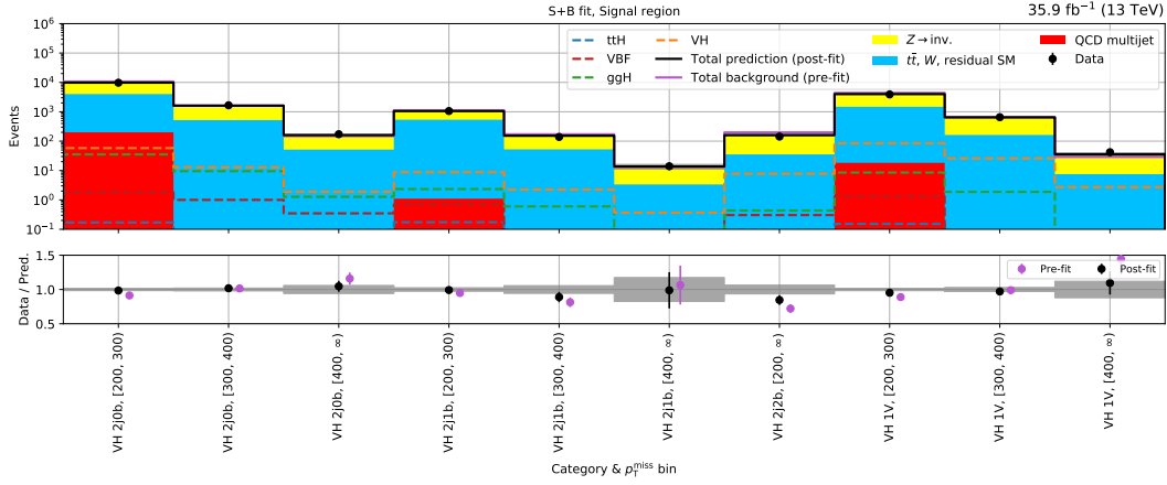
(a) VH —2016
