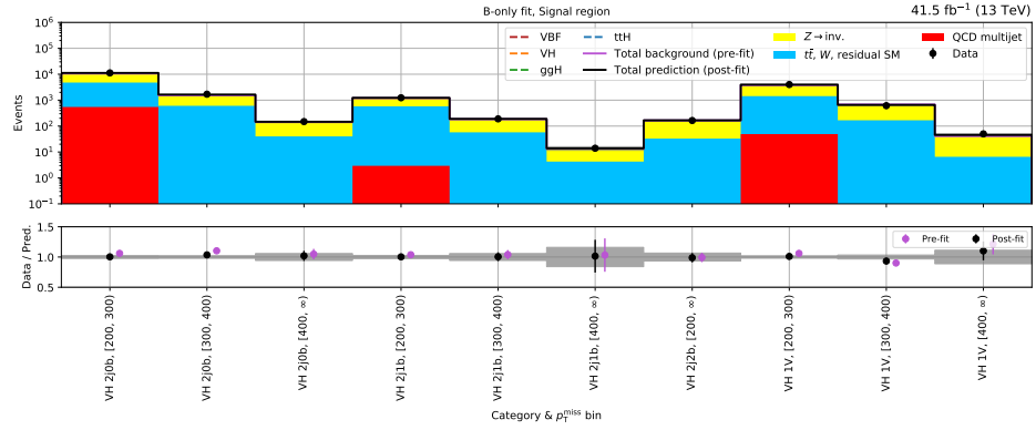
(b) VH — 2017
