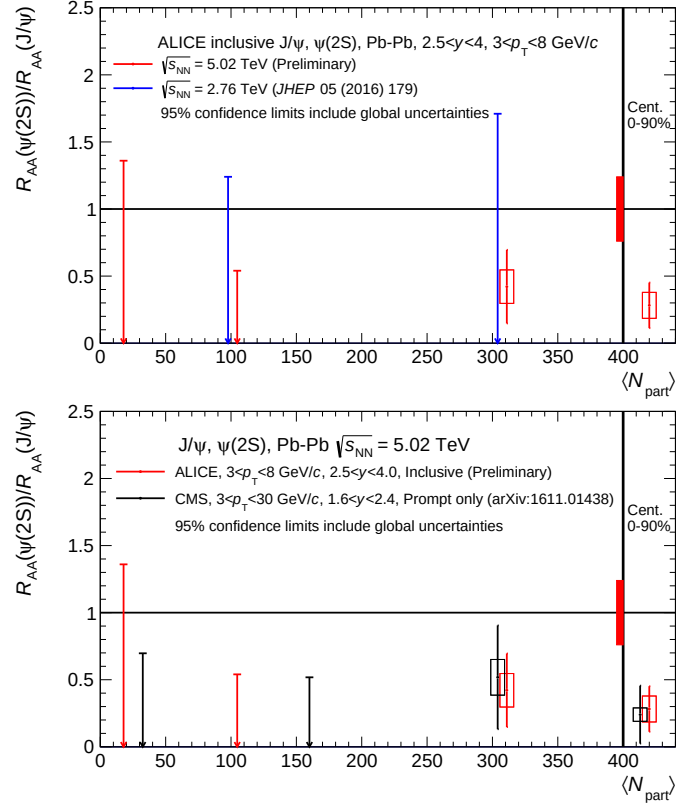
FIGURE 7: Double-rapport R_{AA}^{\psi(2S)}/R_{AA}^{J/\psi} en fonction de N_{part} comparé aux valeurs à \sqrt{s_{NN}} = 2.76 TeV (Haut) et aux valeurs de CMS à \sqrt{s_{NN}} = 5.02 TeV. Pour les intervalles où le signal ne peut pas être extrait, la limite à 95% de confiance est montrée. L'incertitude systématique globale est dessinée autour de l'unité. L'incertitude globale est incluse dans le calcul des intervalles de confiance. La valeur à N_{part} > 400 correspond à la valeur intégrée en centralité (0-90%).
