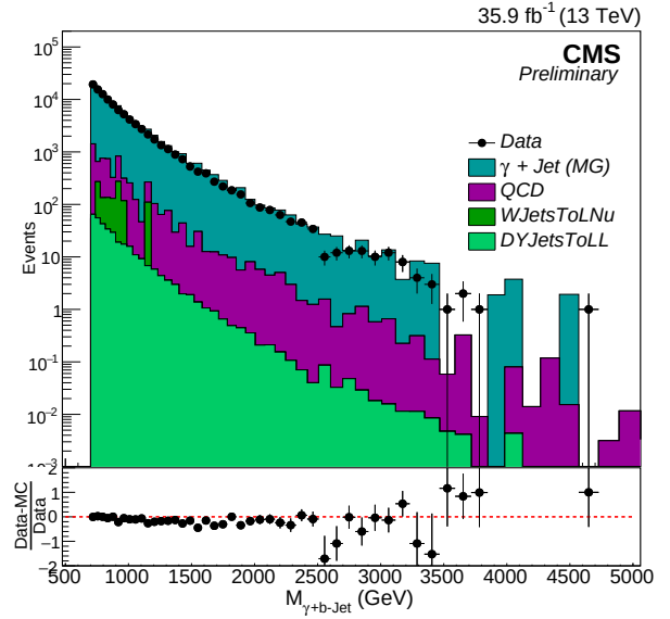
(c) M_{\gamma+\text{jet}} (0 b-tag)
