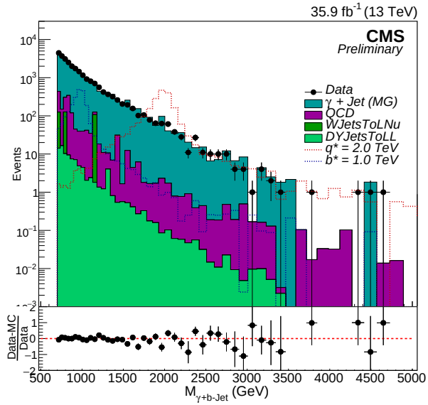
(b) M_{\gamma+\text{jet}} (1 b-tag)
