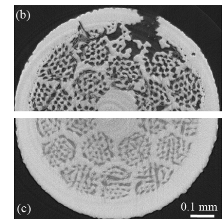
Cette image montre la coupe transversale de deux câbles de Bi-2212. Le câble du bas présente moins de fuites et une porosité nulle grâce à son traitement thermique à une suppression de 100 bars - soit 100 fois la pression utilisée pour produire le câble du haut (images de [Nature Materials, Vol. 13 (2014), 10.1038/nmat3887]).
