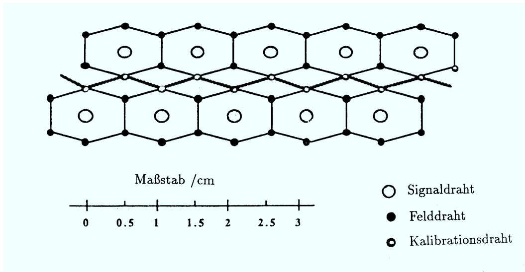
Abbildung 3.3: Aufbau der Driftzellen der ITC
