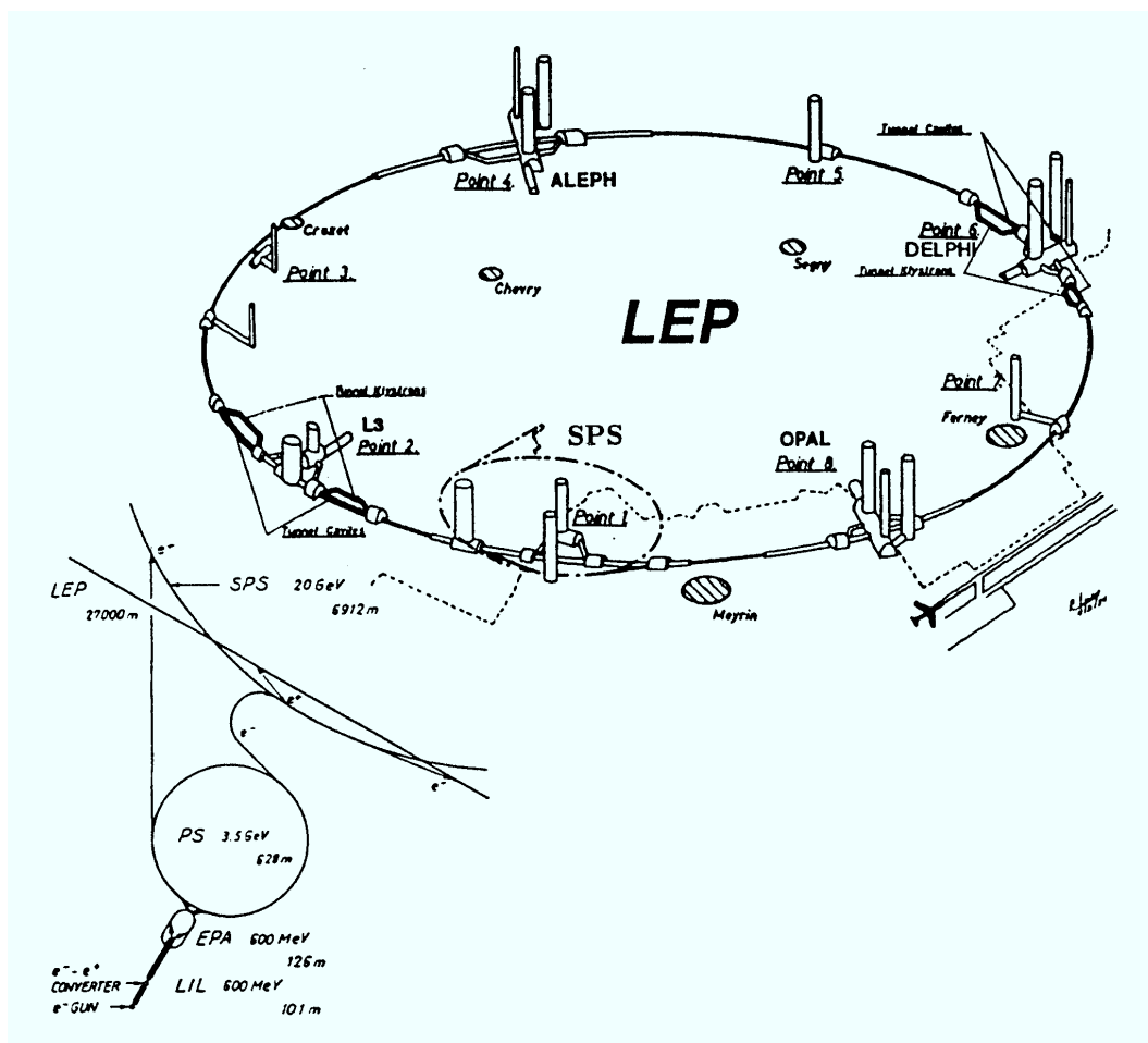
Abbildung 3.1: Speicherring LEP und Injektionskette.
