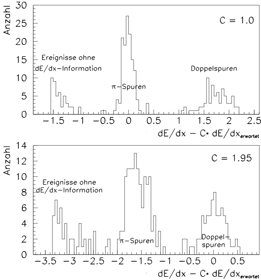
Abbildung 4.5: Doppelspuren: \left(\frac{dE}{dx}\right)_{\text{gemessen}} - C \cdot \left(\frac{dE}{dx}\right)_{\pi} für Spuren in 2-prong Ereignissen. Die Hälfte der Einträge kann überlappenden Spuren zugeordnet werden. (Die Einheit für den Energieverlust ist willkürlich so normiert, das minimalionisierende Teilchen den Wert 1 haben.)
