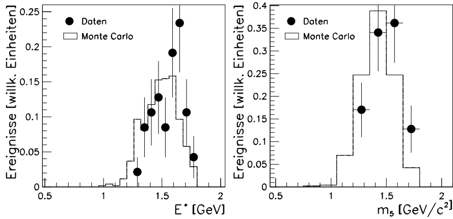
Abbildung 7.9: 5-prong Schnitte: Verteilung von E^* (links) und m_5 für Ereignisse in Schnitt Region I.
