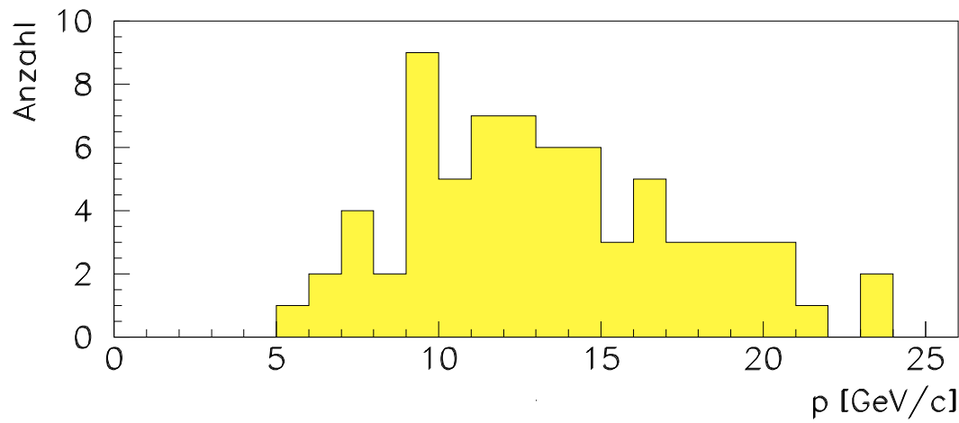
Abbildung 4.6: Impulsspektrum für Doppelspuren aus Ereignissen mit 1-2 Topologie.
