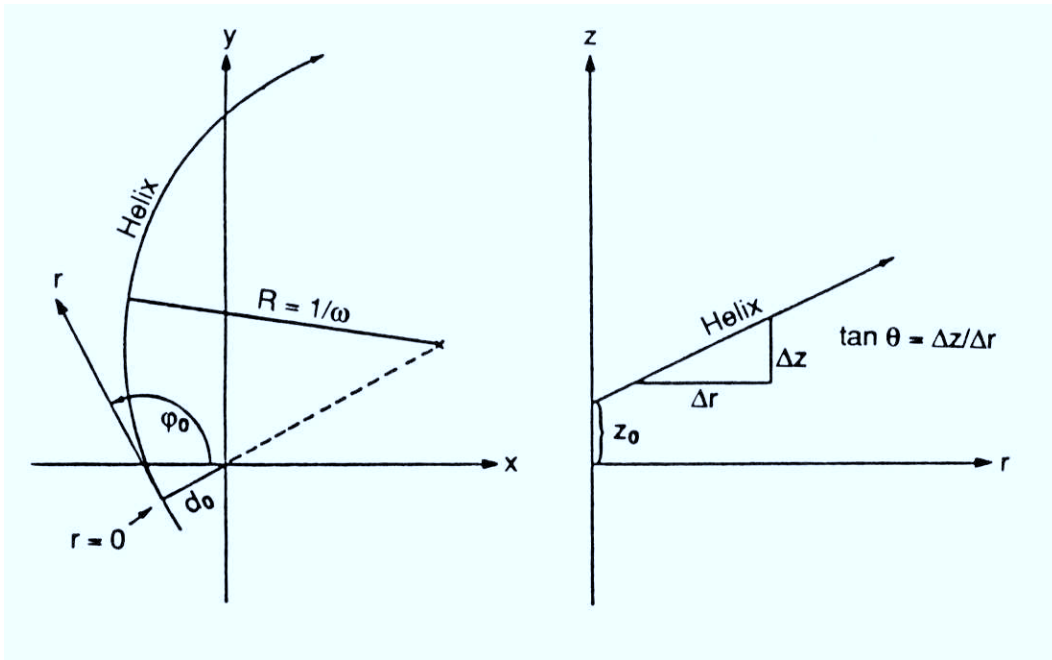
Abbildung 3.6: Helixparameter für Spuren geladener Teilchen
