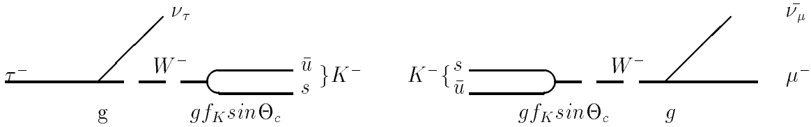
Abbildung 2.4: Feynmangraphen für den Zerfall \tau^- \rightarrow K^- \nu_\tau (links) und K^- \rightarrow \mu^- \nu_\mu (rechts).
