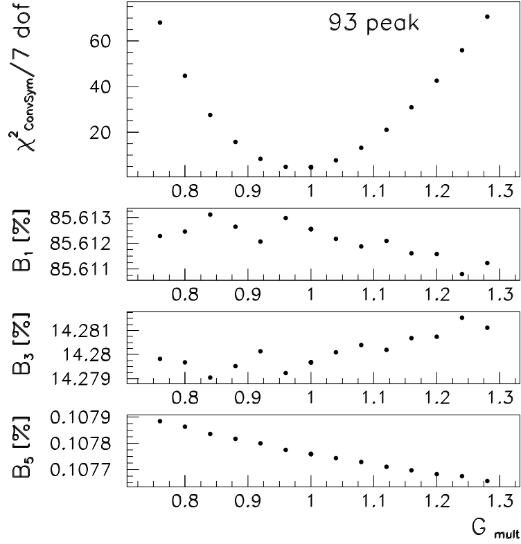
Abbildung 7.10: \chi^2_{SymKonv} als Funktion des variablen Gewichtungsfaktors G_{Konv} von Monte Carlo Ereignissen mit Konversionen am Beispiel der 1993 auf dem Resonanz-Peak aufgenommenen Daten. Darunter: Topologische Verzweungsverhältnisse B_i ( i=1,3,5 ) als Funktion von G_{Konv} .
