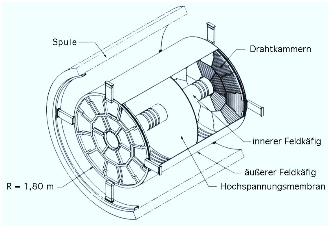
Abbildung 3.4: Aufbau der Zeitprojektionskammer (TPC)
