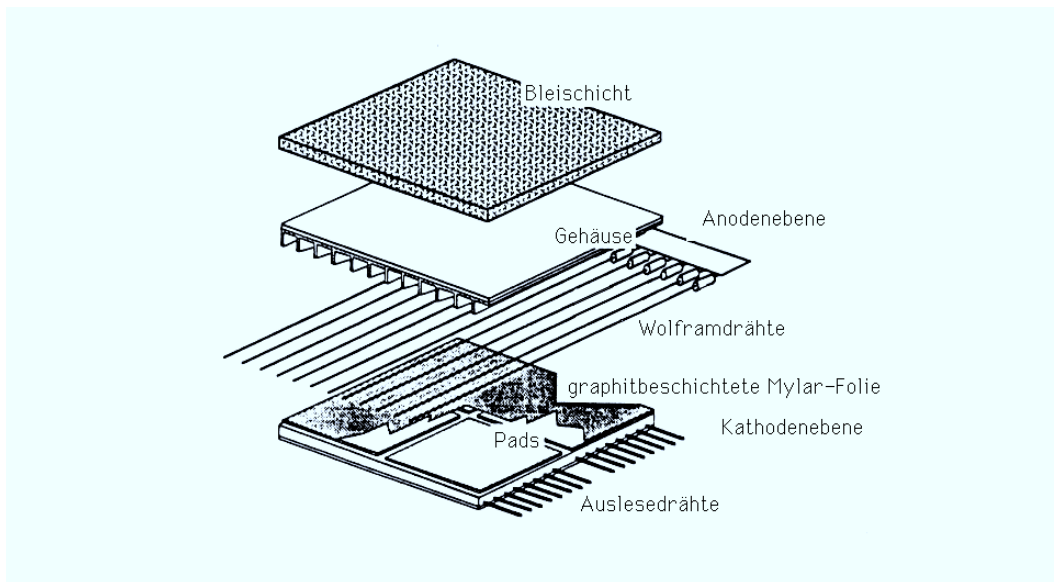
Abbildung 3.8: Aufbau der Proportionalkammern in einer typischen ECAL-Schicht
