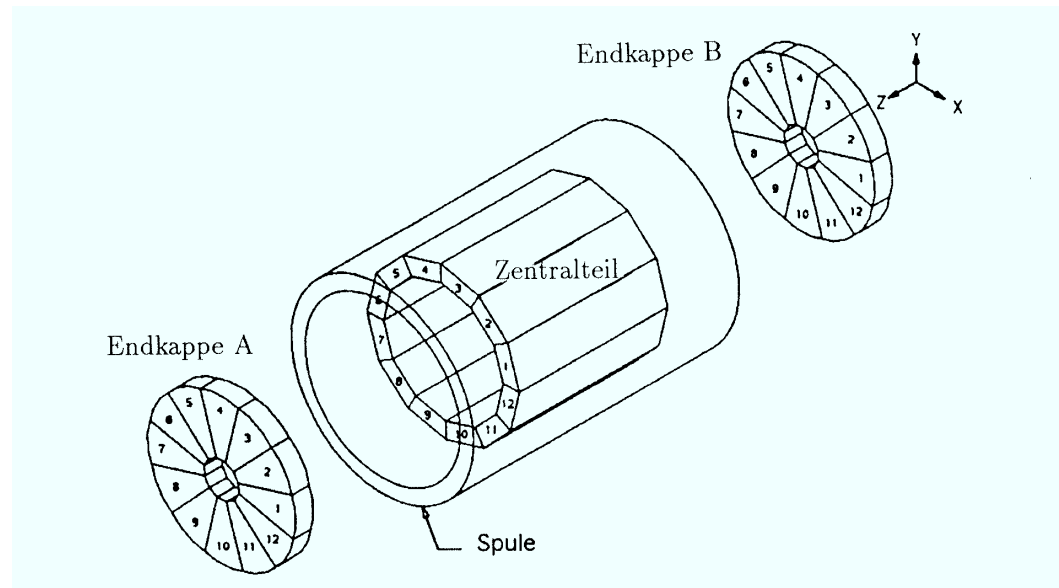
Abbildung 3.7: Aufbau des elektromagnetischen Kalorimeters (ECAL)
