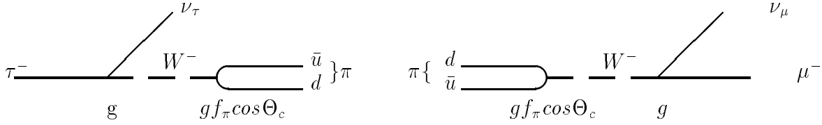
Abbildung 2.3: Feynmangraphen für den Zerfall \tau^- \rightarrow \pi^- \nu_\tau (links) und \pi^- \rightarrow \mu^- \nu_\mu (rechts).
