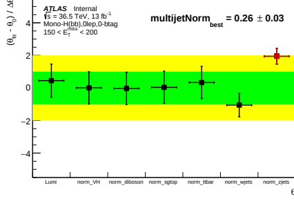
(a) 0-btag, 150 \text{ GeV} < E_T^{\text{miss}} < 200 \text{ GeV}
