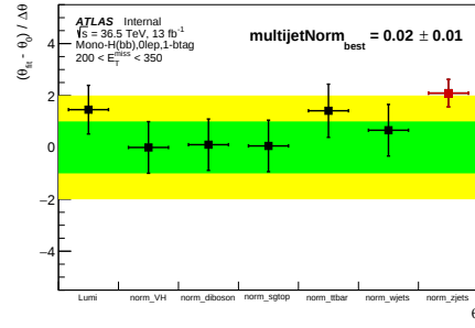
(d) 1-btag, 200 \text{ GeV} < E_T^{\text{miss}} < 350 \text{ GeV}
