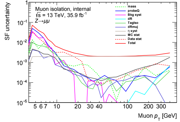
(d) GradientLoose
