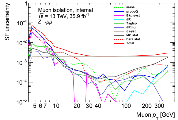
(f) Gradient
