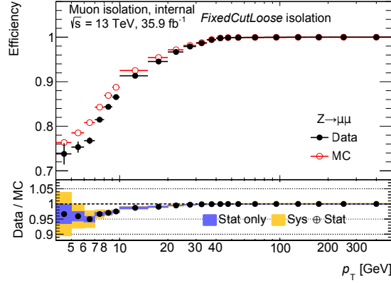
FIGURE E.1 – Efficacités (haut) et facteurs d’échelle (bas) du point de fonctionnement FixedCutLoose . Les données sont en noir et la simulation est en rouge. Les incertitudes statistiques seules (violet) et avec les systématiques (jaune) des facteurs d’échelle sont représentées par les plages de couleur.
