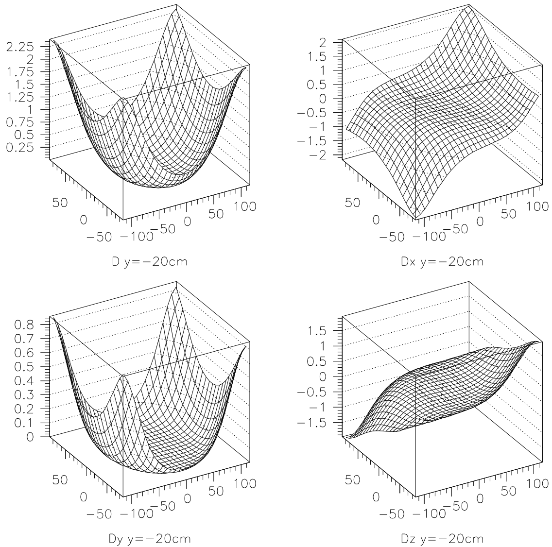
Abbildung 3.19 Korrekturen in einer Ebene bei y = -20 cm. Nach oben sind die Korrekturen, nach links die x-Koordinate und nach rechts die z-Koordinate aufgetragen. Alle Angaben in cm.
