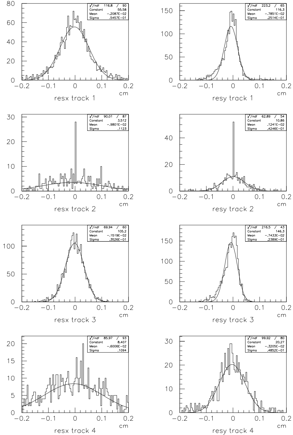
Abbildung 4.24 Gemessene Residualverteilungen aller vier Spuren für den Run 446 mit elektrischen Verzerrungskorrekturen ( \theta=5.4^\circ , B=0\text{T} , 20 Ereignisse, \text{NeCO}_2 )
