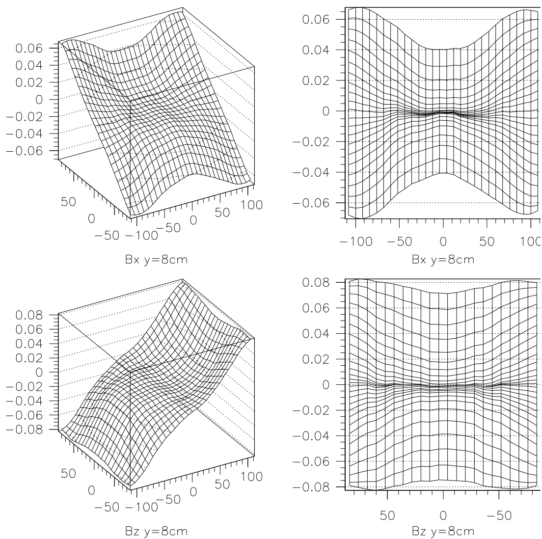
Abbildung 3.8 NebenkompONENTEN des gemessenen Magnetfeldes in einer Ebene ( y=8 \text{ cm} ) mit einer Projektion zur Verdeutlichung von Verzerrungen
