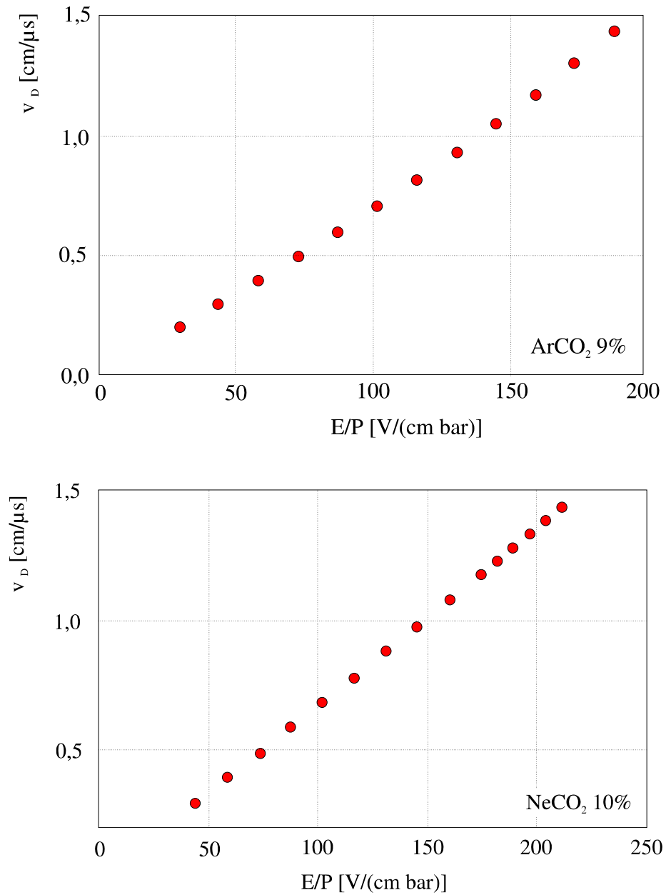
Abbildung 3.6 Driftgeschwindigkeit als Funktion des reduzierten elektrischen Feld für die beiden Gasmischungen \text{ArCO}_2 (9%) und \text{NeCO}_2 (10%)
