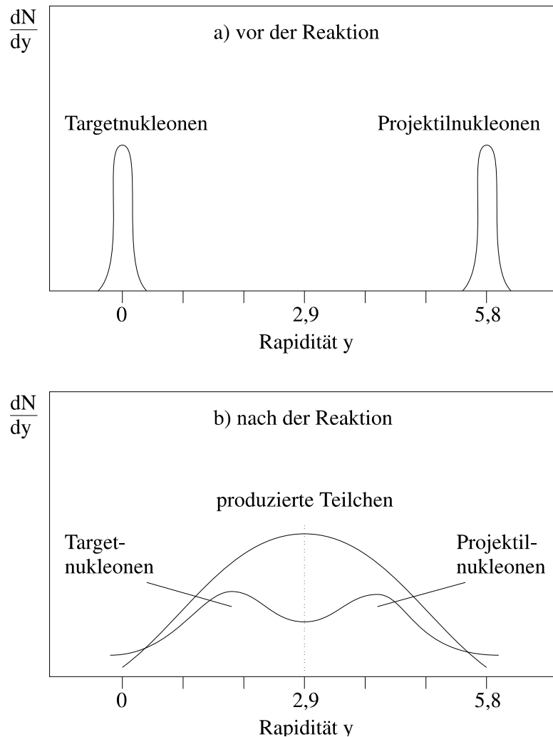
Abbildung 1.3 Rapidityverteilung vor (a) und nach (b) der Reaktion
