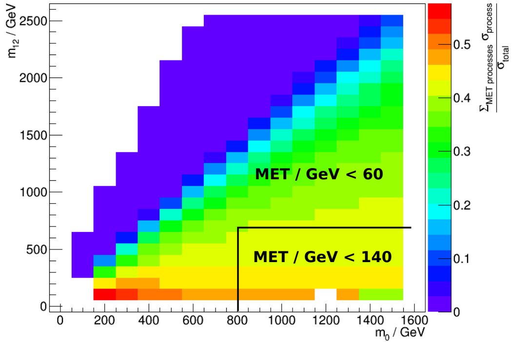
Abbildung 3.13.: Die Anteile der verschiedenen Prozesse relativ zum Gesamtwirkungsquerschnitt, abhängig von den mSUGRA Parametern m_0 und m_{12} . Oben (a) für den Zerfallskanal aus Abb. 1.1, unten (b) die Summe der relativen Anteile der Prozesse aus Abb. 3.10.
