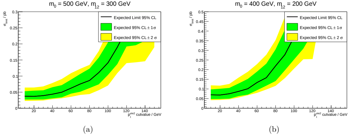
Abbildung 3.17.: Das expected Limit gegen den p_T^{ele2} Selektionsparameter für ausgewählte Signalfunkte.
