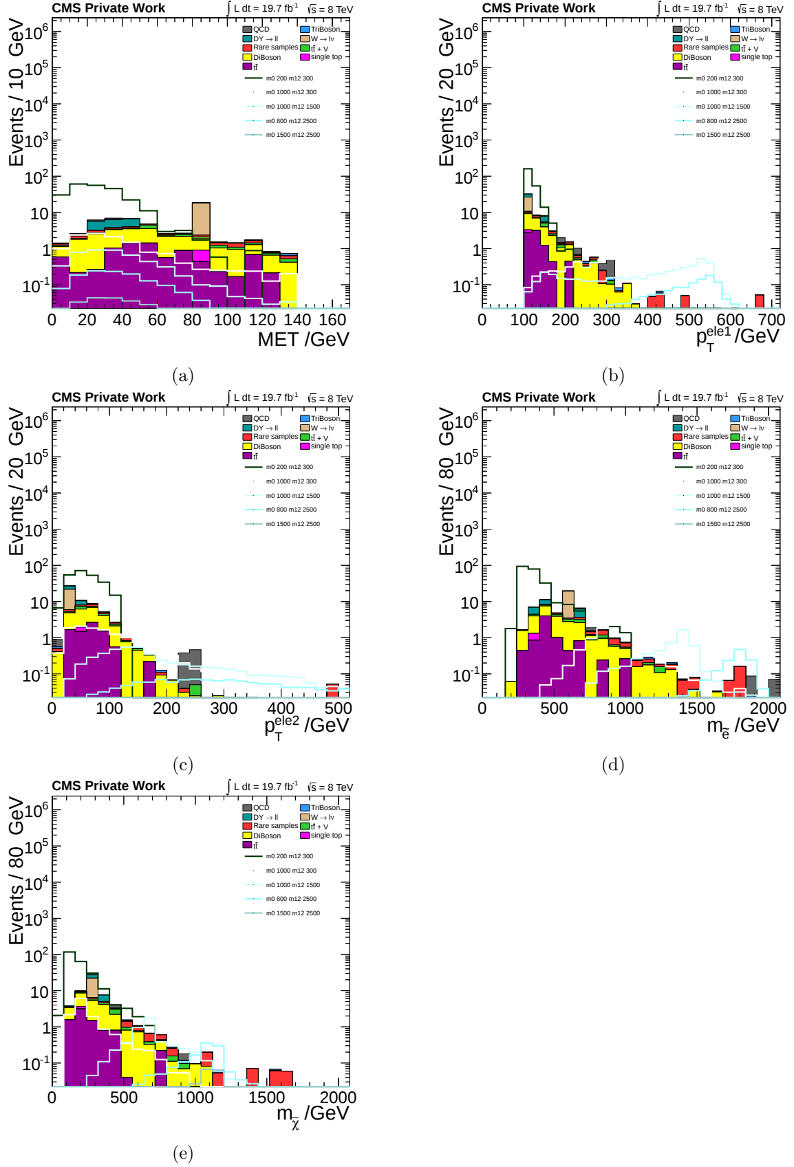
Abbildung 4.2.: Die finalen Verteilungen der fehlenden Transversalenergie (a), der transversalen Impulse der Elektronen (b) & (c) und der rekonstruierten Selekttron- (d) und Gauginomasse (e).
