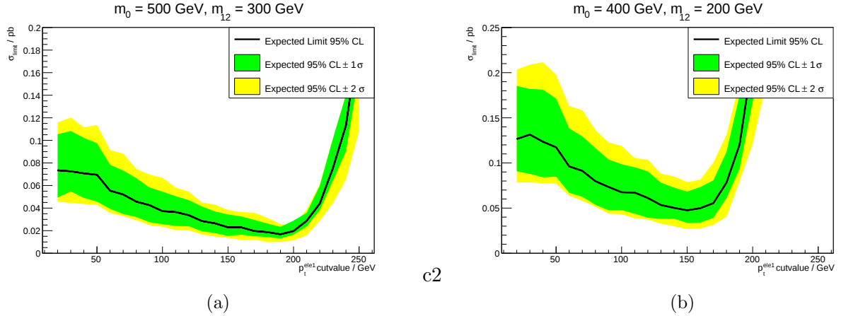
Abbildung 3.14.: Das expected Limit gegen den p_T^{ele1} Selektionsparameter für ausgewählte Signalpunkte.
