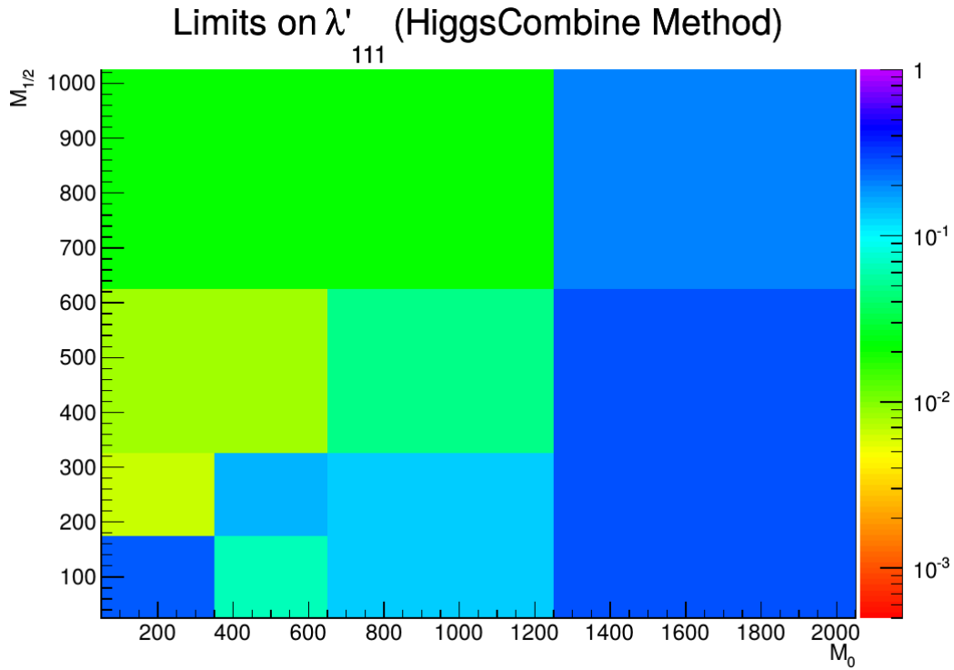
Abbildung 1.3.: Bisherige Limits (95% C.L.) auf resonante Selektionproduktion durch die Kopplung \lambda'_{111} , entnommen aus [9]. Oben (a) die Limits aus netrinolosem Doppelbetazerfall, unten (b) die möglichen Limits mit CMS Daten aus einer Studie von 2011. Die mSUGRA Parameter sind A_0 = 0 , \tan(\beta) = 20 und \text{sign}(\mu) = +1 .
