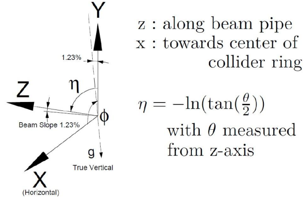
Abbildung 2.2.: Das in CMS verwendete Koordinatensystem, entnommen aus [10].
