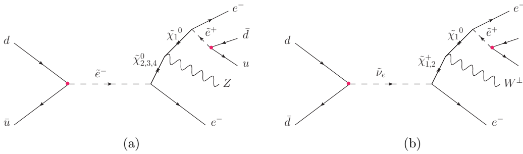
Abbildung 3.10.: Feynman Diagramm des Selektion Zerfalls \tilde{e}^- \rightarrow 2e + 2jet + Z (a) und des Sneutrino Zerfalls \tilde{\nu}_e \rightarrow 2e + 2jet + W (b). Beide Prozesse können die Signalsignatur und MET erzeugen. An den roten Vertices ist die R Parität verletzt.
