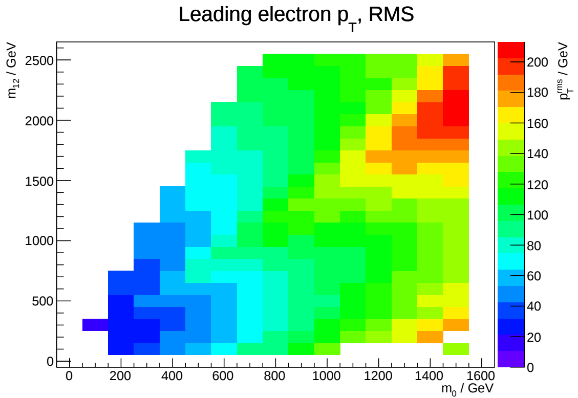
Abbildung 3.15.: Der Mittelwert und Breite der Verteilung des transversalen Impulses des härteren Elektrons ( p_T^{\text{ele1}} ).
