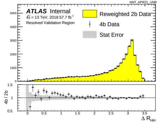
(d) After Reweighting
