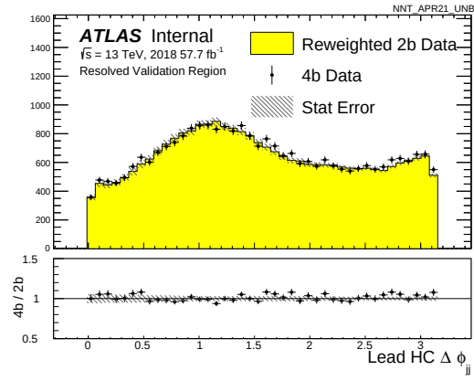
(d) After Reweighting
