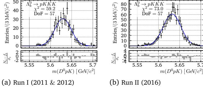
Fig. I.11.: Fit to \Lambda_b^0 \rightarrow pK K K MC in m(D^0 p K)
