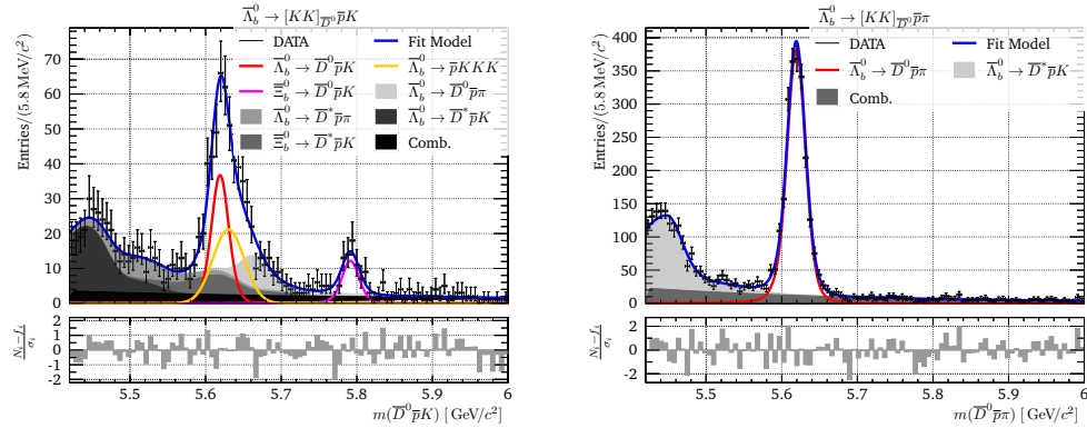
(d) \bar{\Lambda}_b^0 -type - m(D^0 \bar{p} h^+) , with D^0 \rightarrow K K
