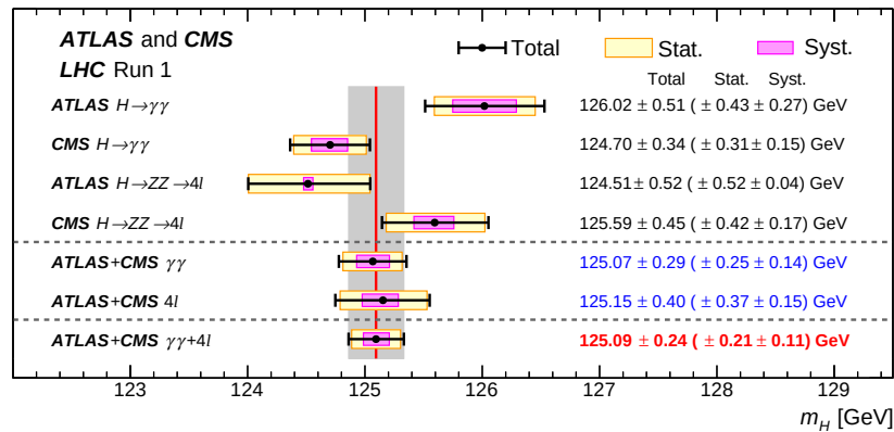
Figure 1: Résumé des mesures de masse du boson de Higgs à partir des analyses individuelles d'ATLAS et de CMS et de l'analyse combinée utilisant les données de 25 \text{ fb}^{-1} du Run 1 [3].
