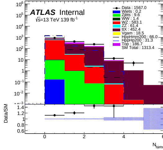
(d) N_{b\text{jets}} distribution (Log Scale)
