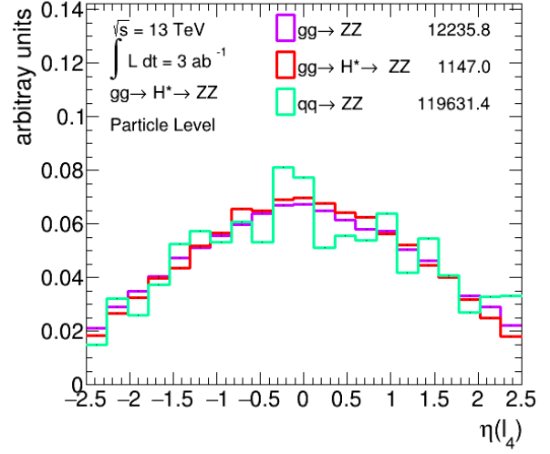
(d) \eta(l_4)
