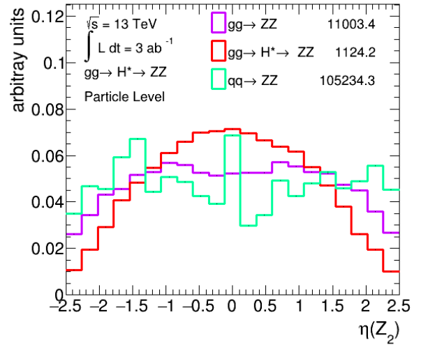
(d) \eta(Z_2)
