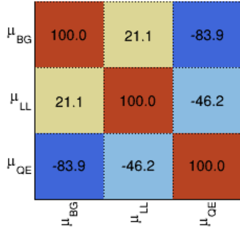
(d) Background scaling 0.25
