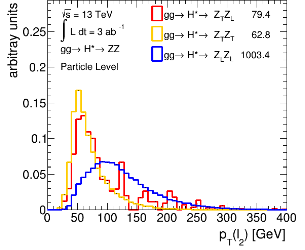
(b) p_T(\ell_2)
