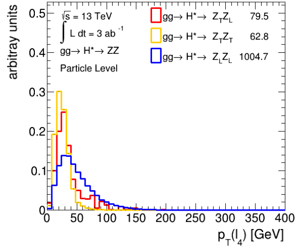
(d) p_T(\ell_4)
