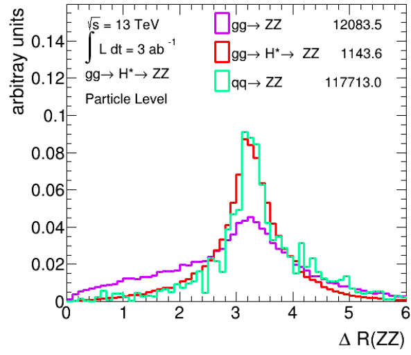
(c) \Delta R(ZZ)
