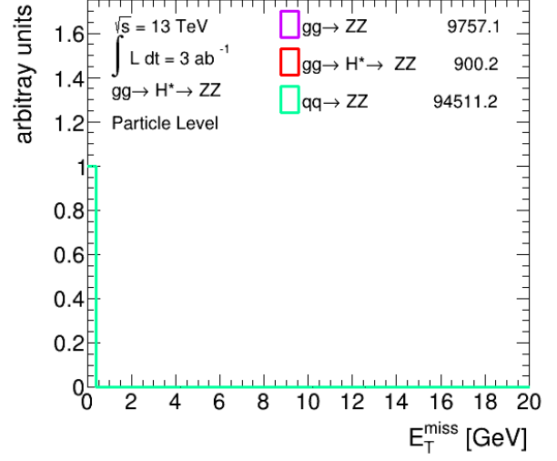
(b) E_T^{\text{miss}}
