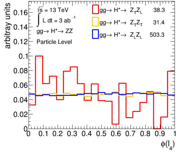
(d) \phi(\ell_4)
