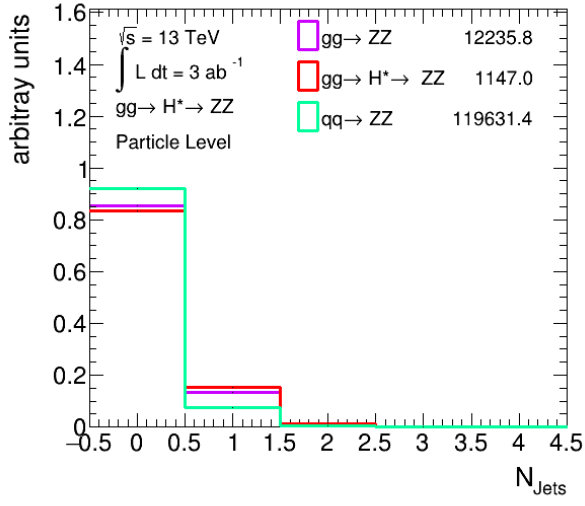
(a) N_{jets}
