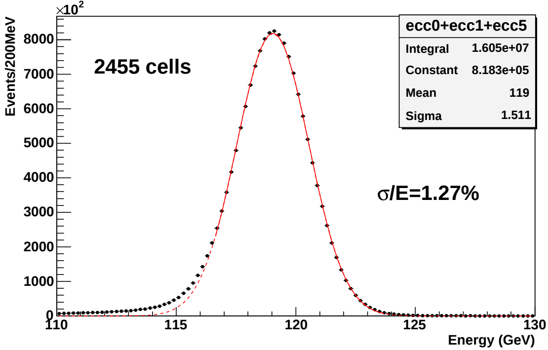
FIGURE 4.37 – Spectre en énergie total pour les électrons de 119 GeV collectés sur les trois modules. Le résultat de l'ajustement gaussien démarrant à -1.5\sigma de la valeur moyenne est superposé sur la distribution.
